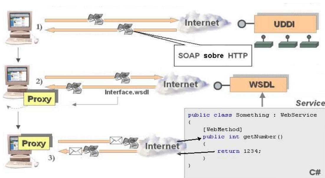
Figura 7 – Secuencia de llamada de Web Services usando C#
