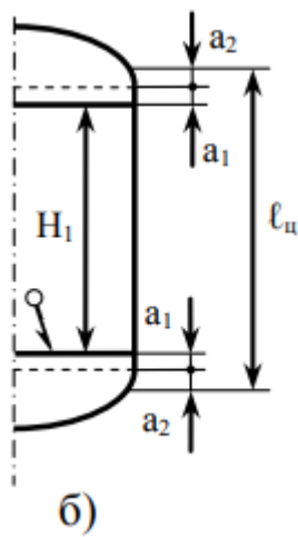
Рисунок 1 – Схемы к определению расчетной длины цилиндрической оболочки l_{\text{ц}} для корпуса 10.
