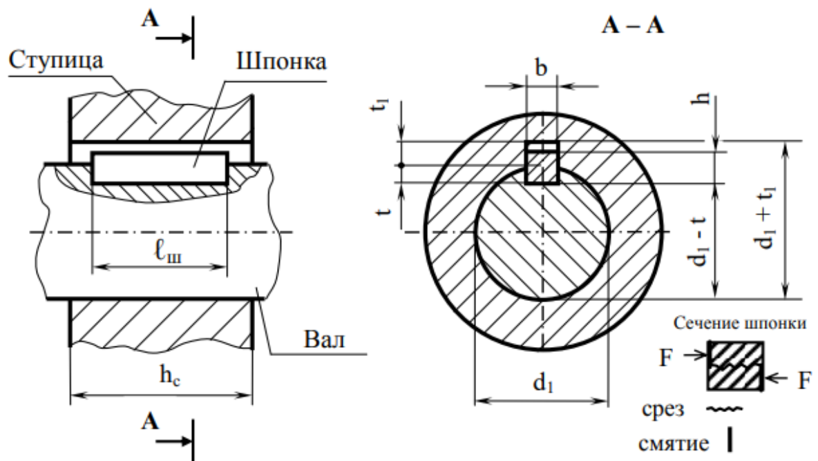
Рисунок 4 – Схема к расчету шпоночного соединения
