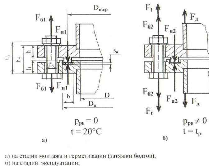
Рисунок 2 – Расчетная схема фланцевого соединения.
