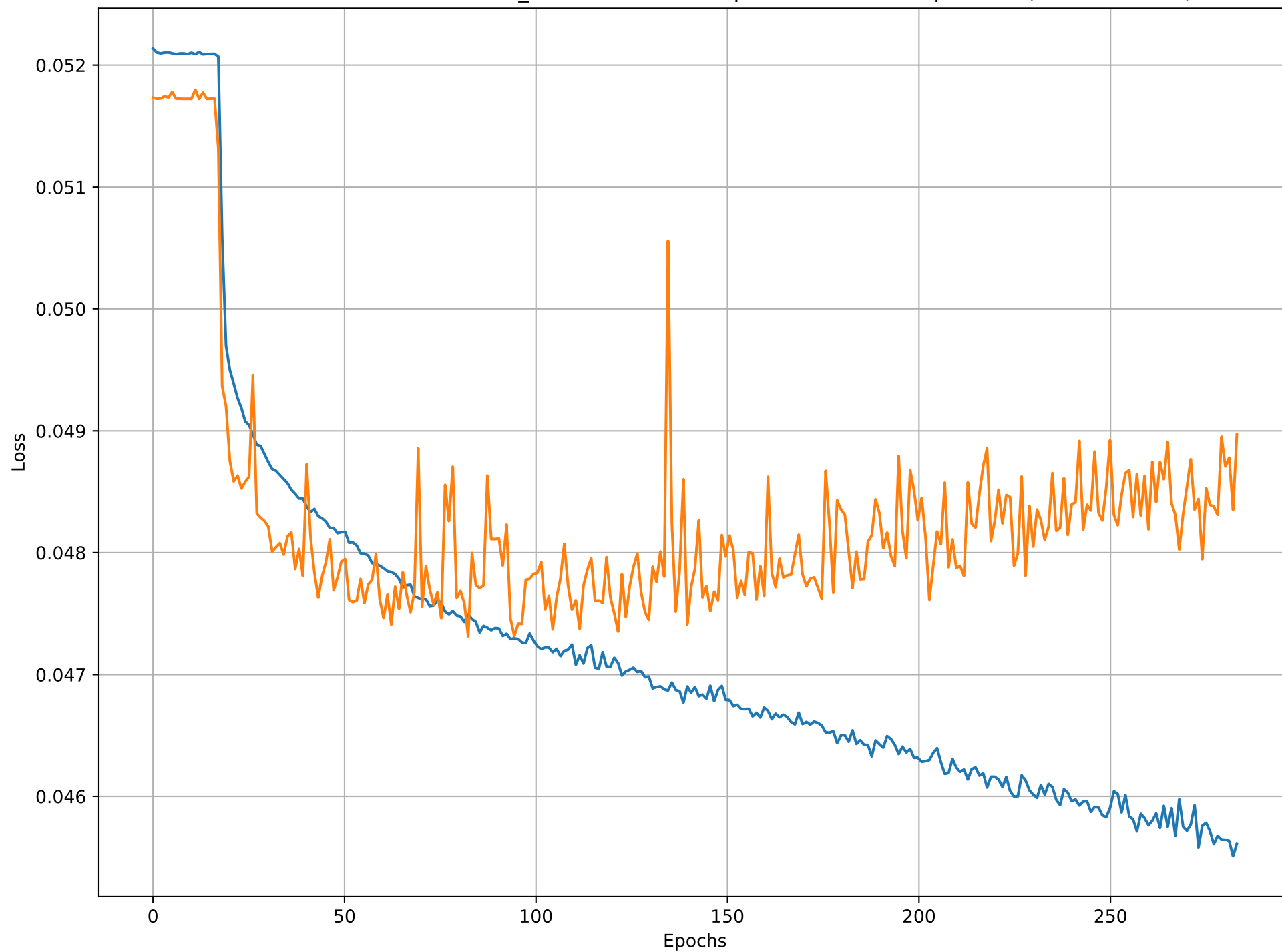
Evolution de loss et validation_loss au cours des epochs. Validation split=0.4 (score=0.0473)
