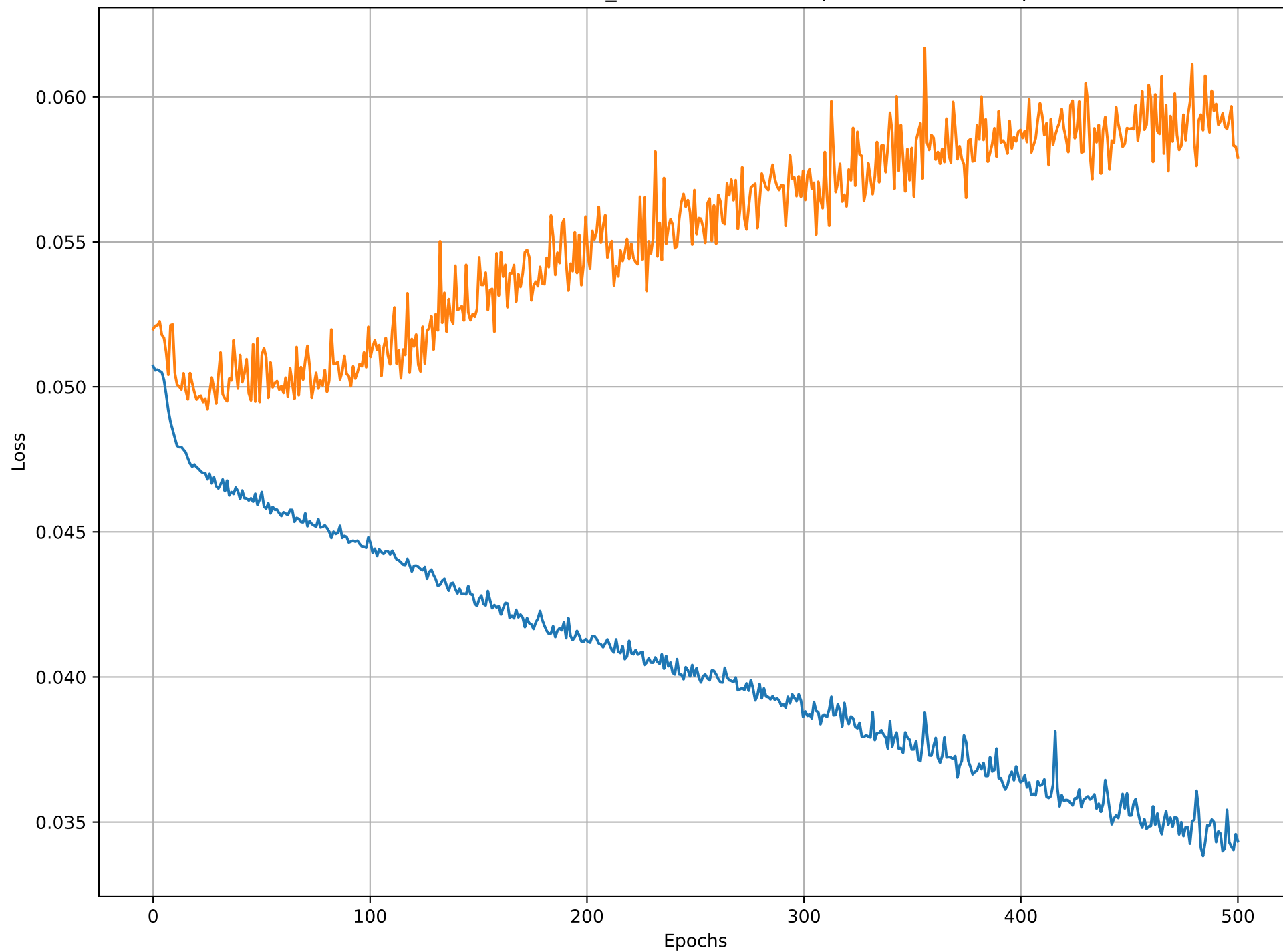
Evolution de loss et validation_loss au cours des epochs. Validation split=0.4
