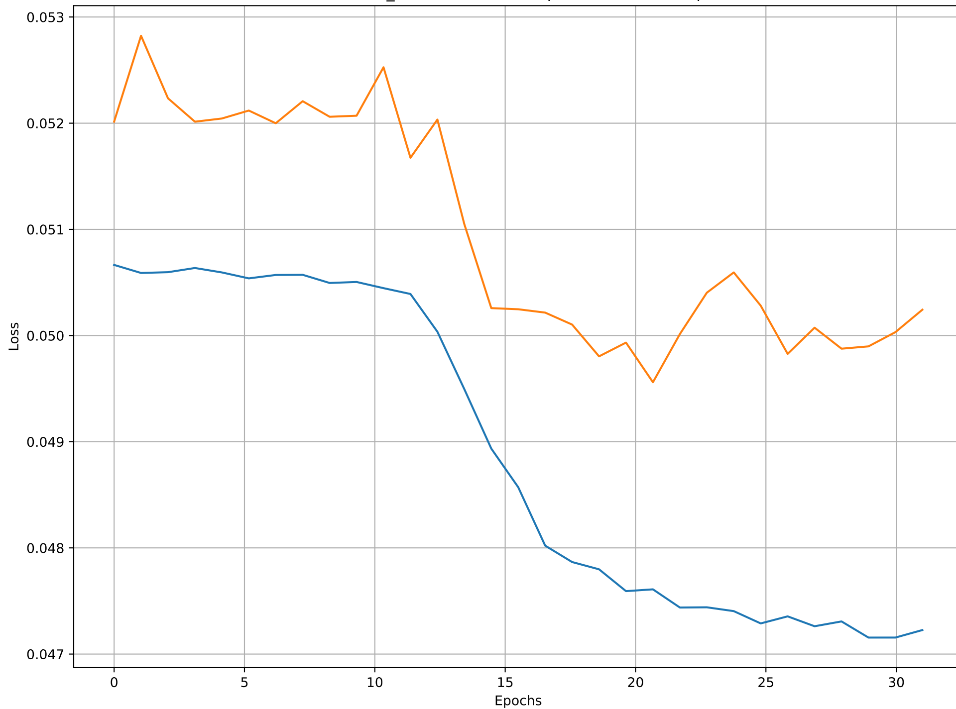
Evolution de loss et validation_loss au cours des epochs. Validation split=0.4 (score=0.0496)
