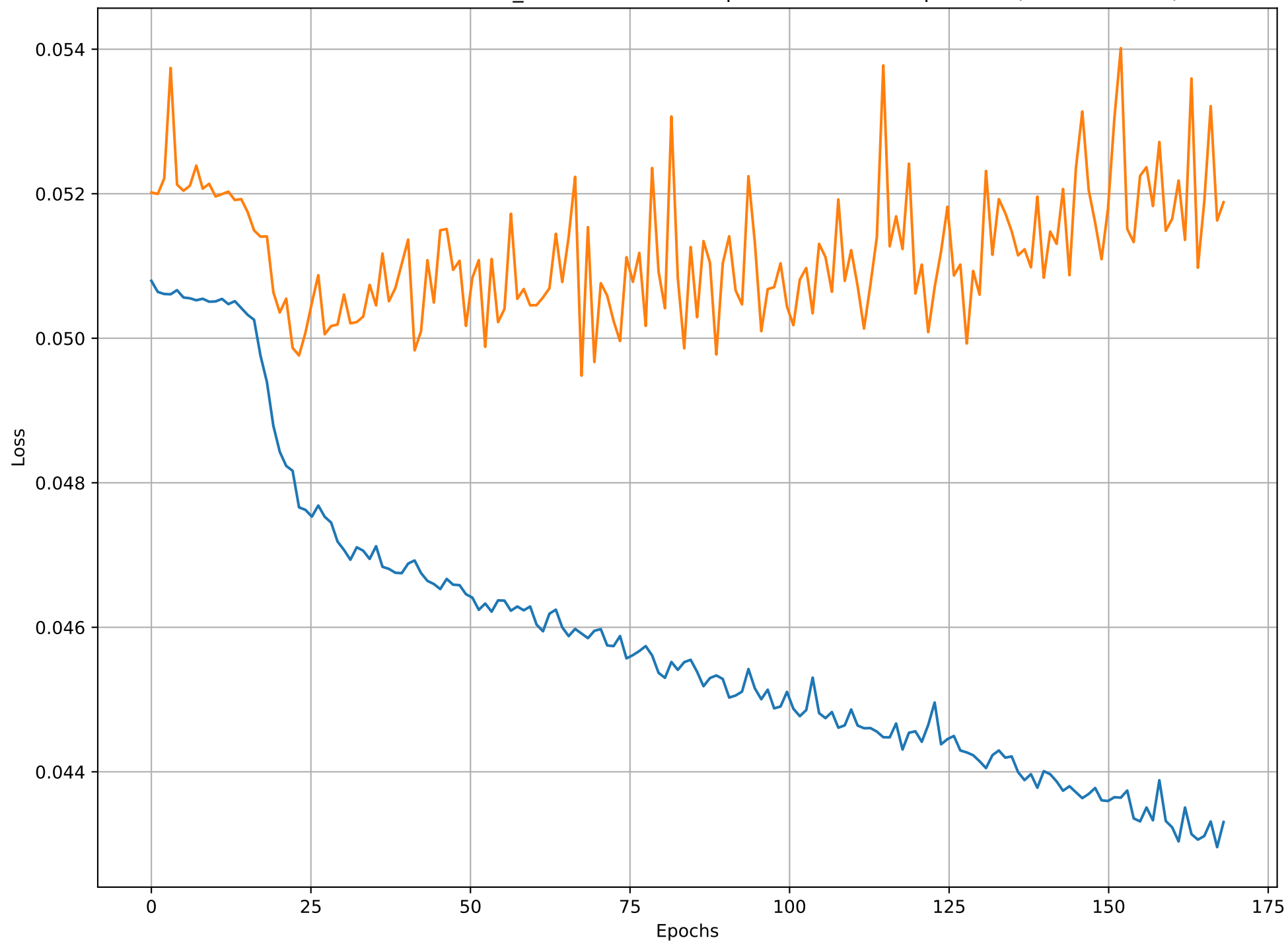
Evolution de loss et validation_loss au cours des epochs. Validation split=0.4 (score=0.0495)
