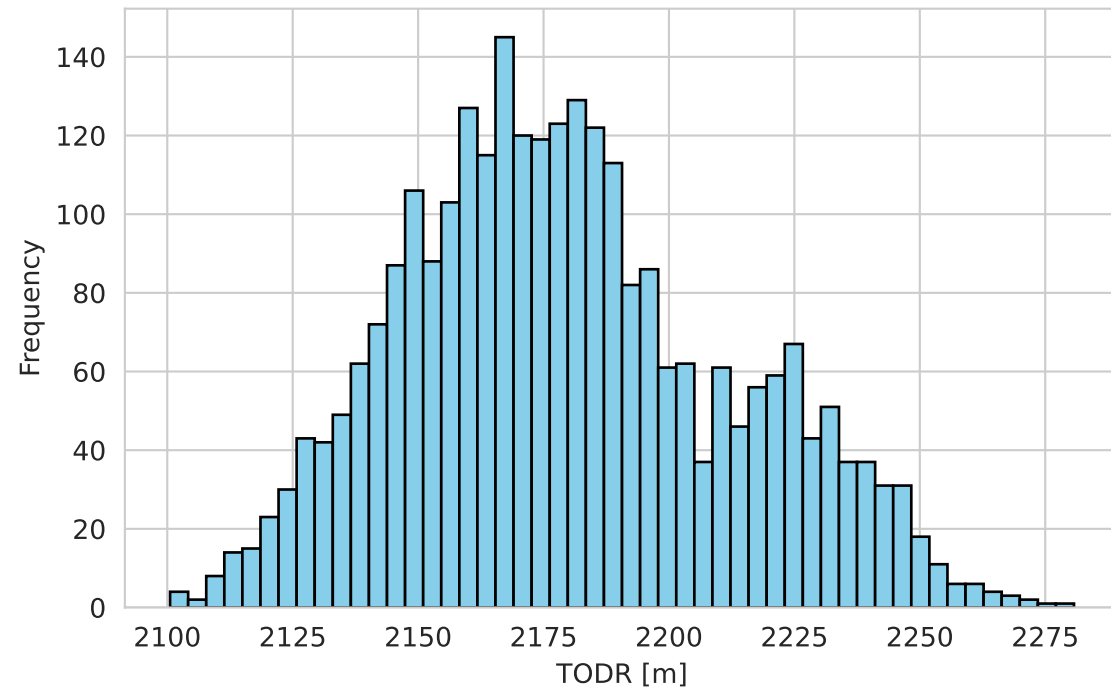
SSP585 Scenario
