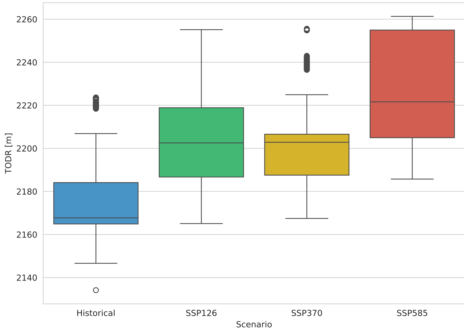
TODR (JJA) A320 - V2500-A1 - EBBR - QDM
