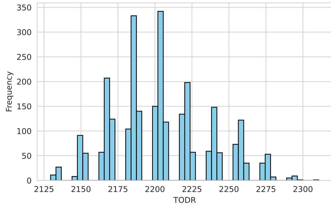
SSP585 Scenario
