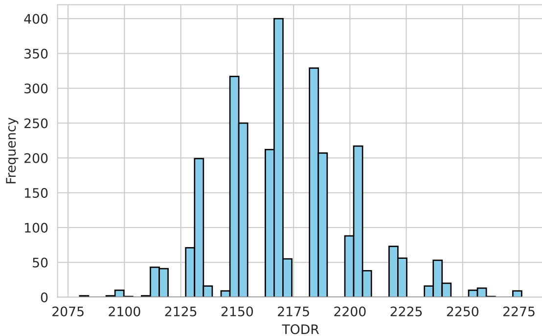
SSP370 Scenario
