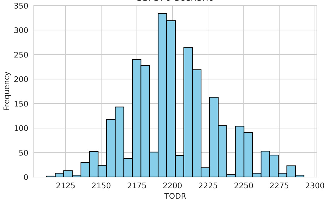
SSP370 Scenario
