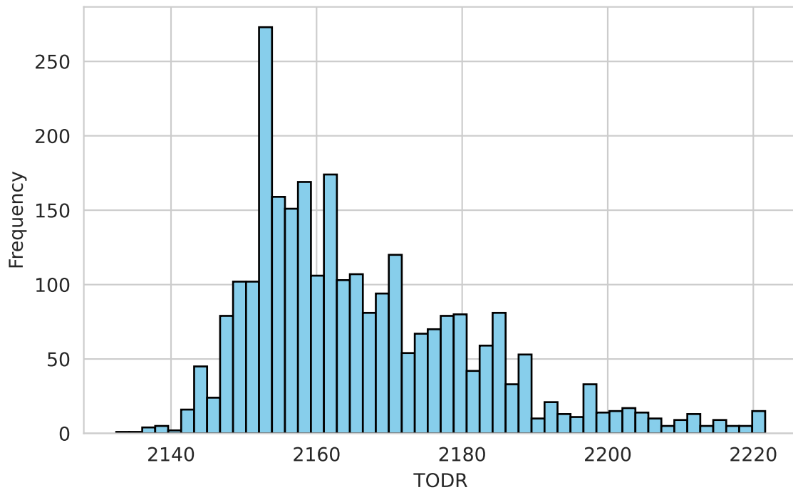
SSP370 Scenario
