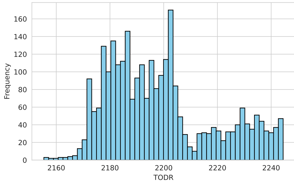
SSP585 Scenario
