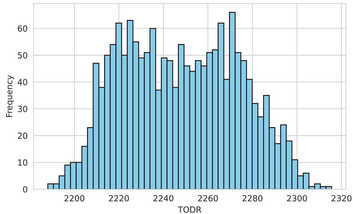
SSP585 Scenario
