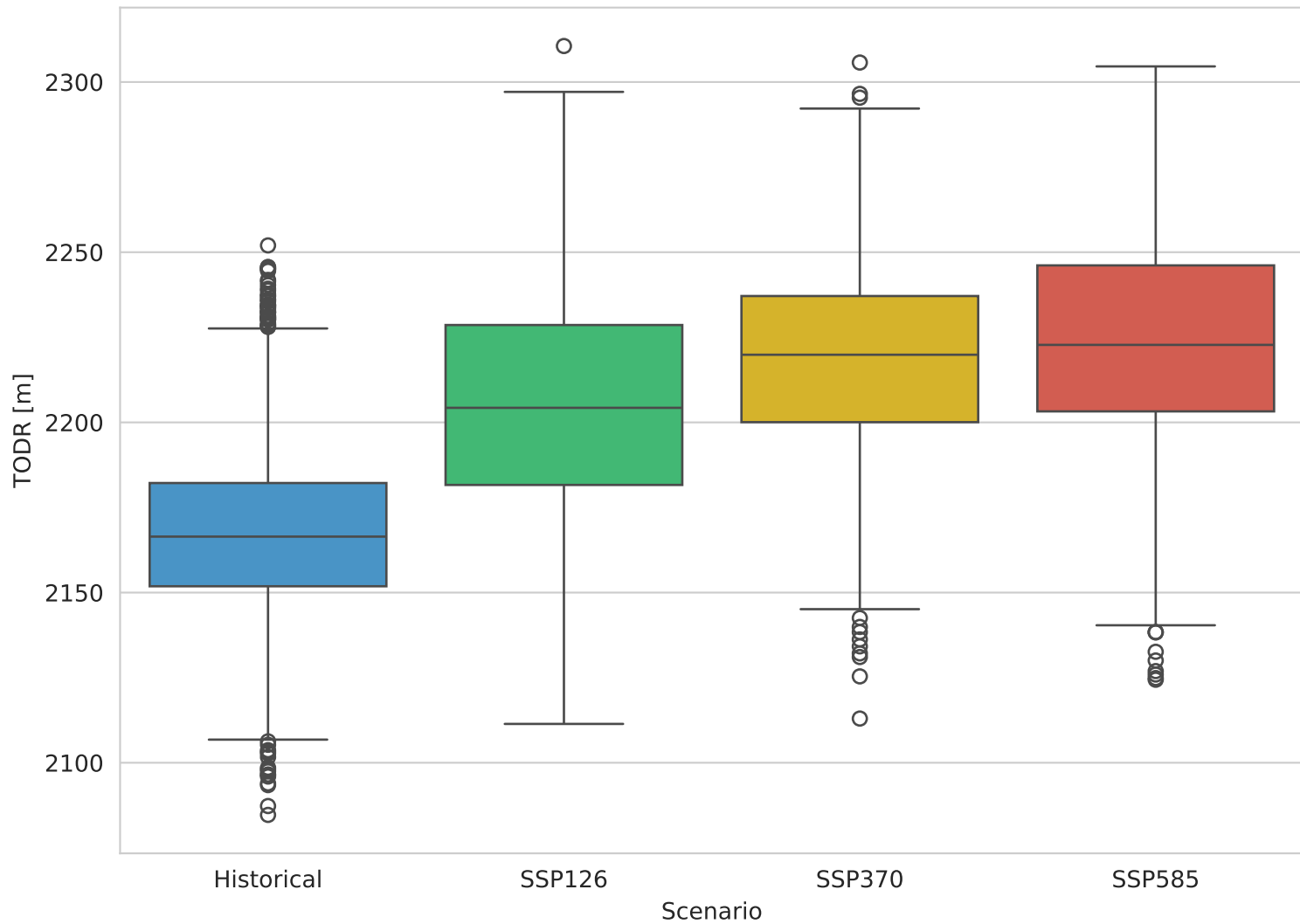
TODR (JJA) A320 - V2500-A1 - EGLL - NOQDM
