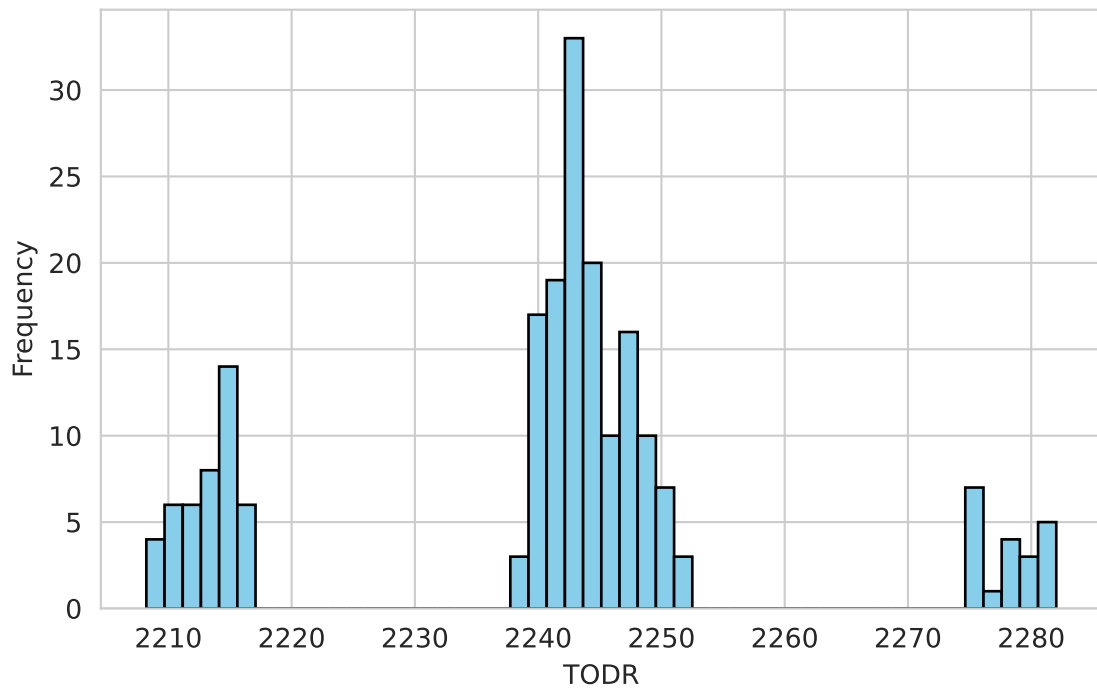
SSP370 Scenario
