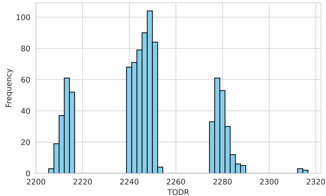
SSP585 Scenario
