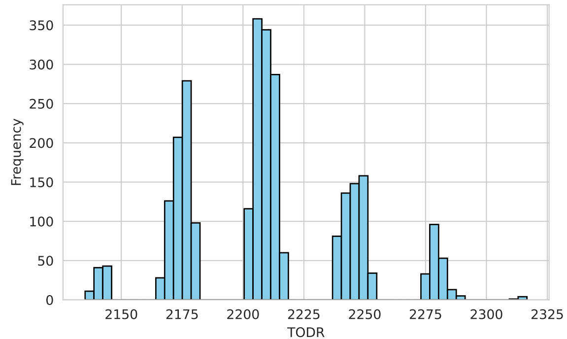
SSP585 Scenario
