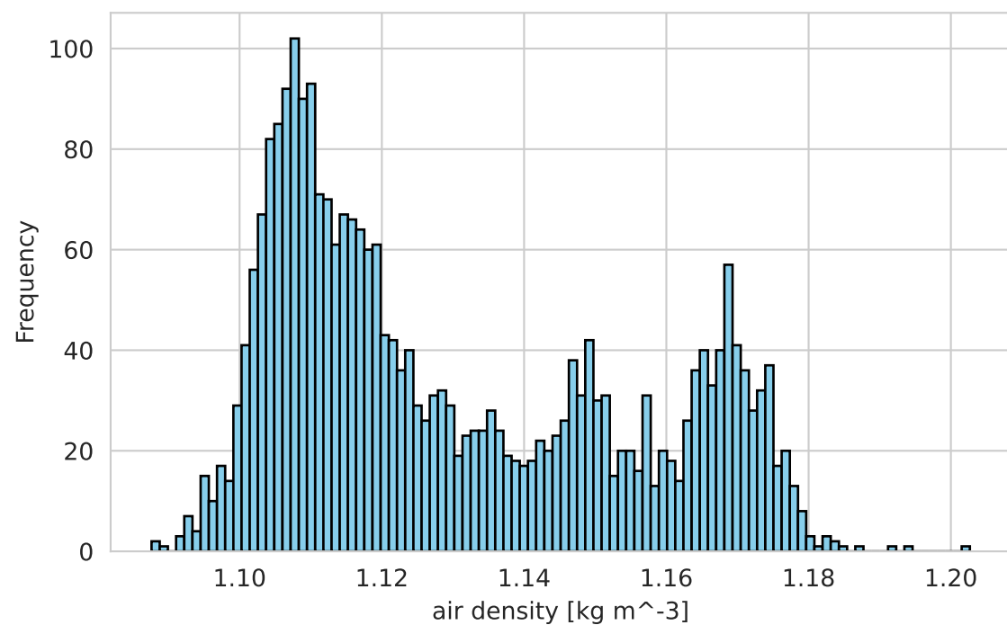
SSP585 Scenario
