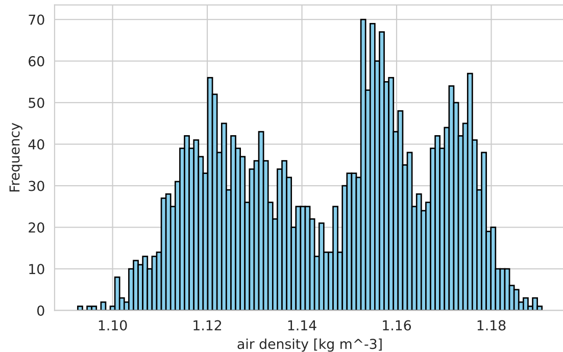
SSP585 Scenario
