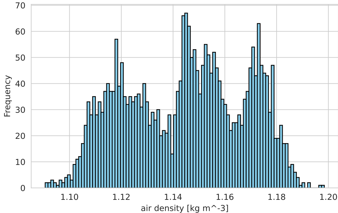
SSP370 Scenario
