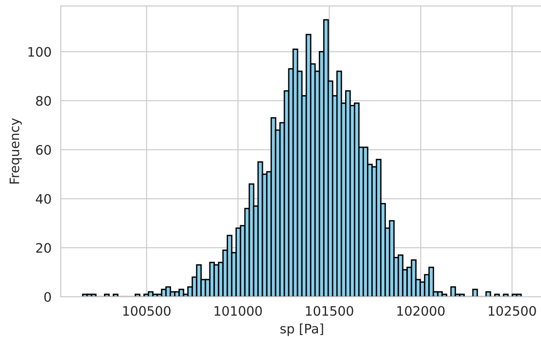
SSP585 Scenario
