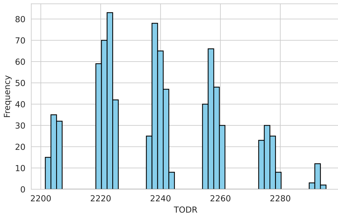
SSP370 Scenario
