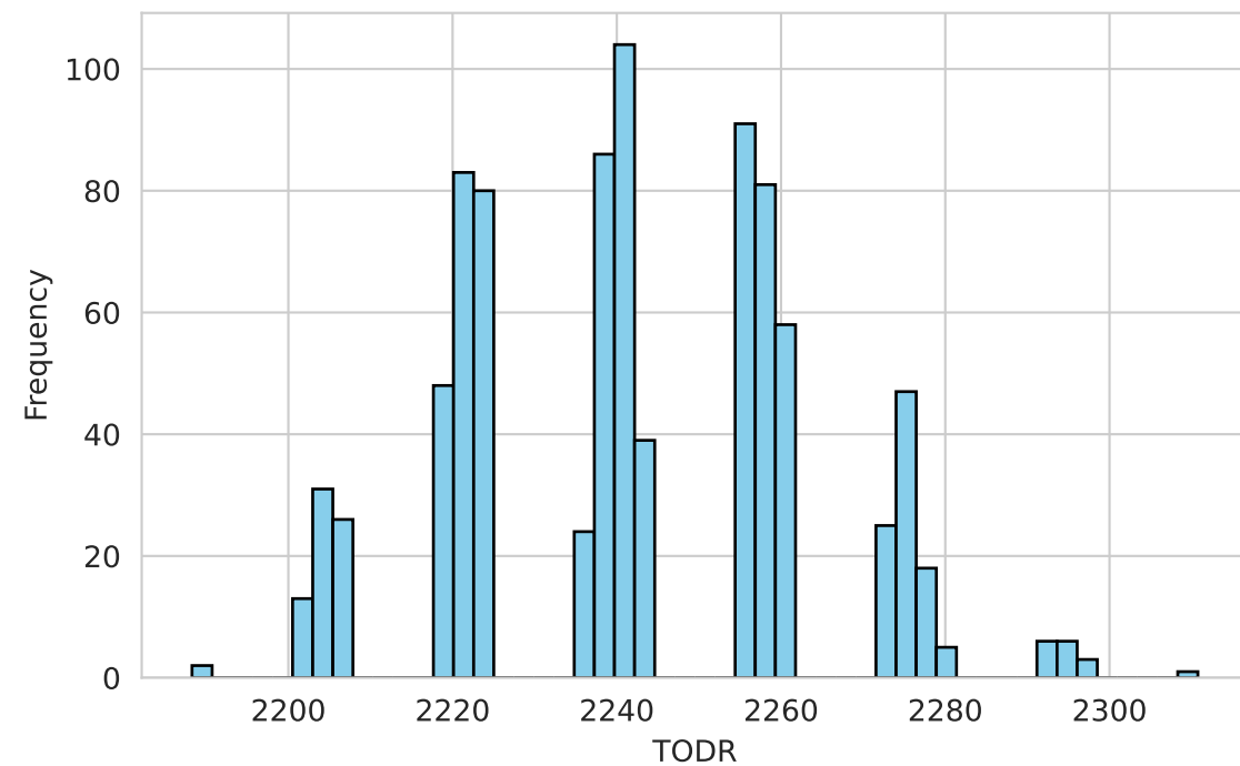
SSP126 Scenario
