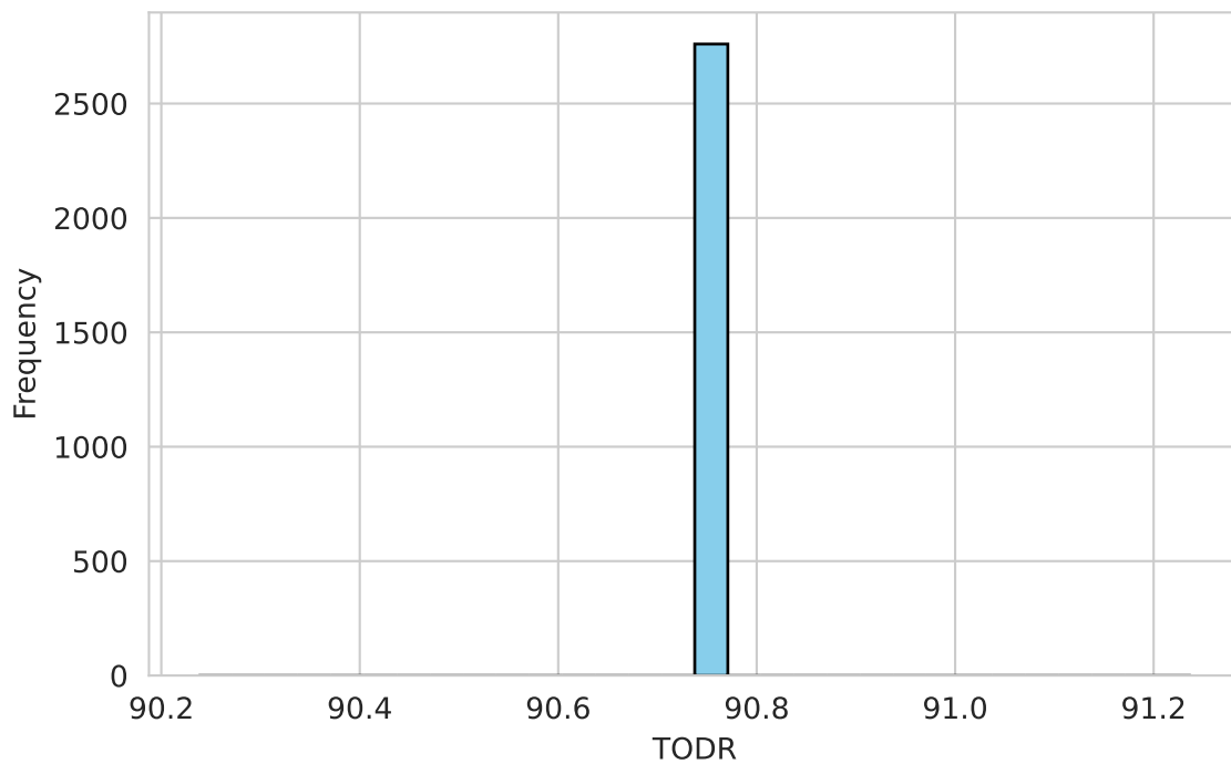
SSP370 Scenario
