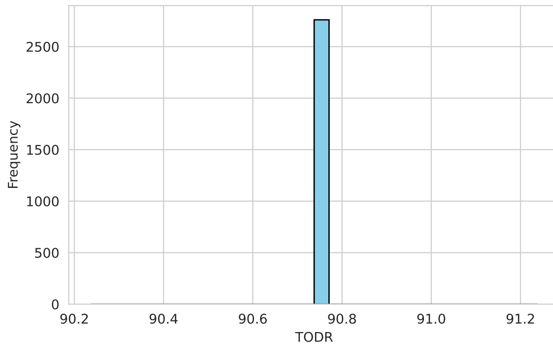
SSP585 Scenario
