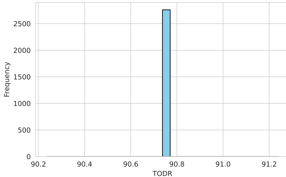
SSP126 Scenario
