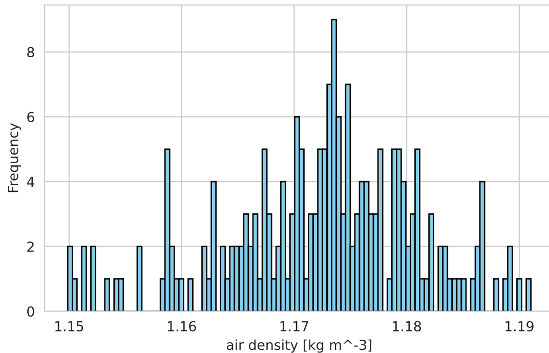
SSP370 Scenario
