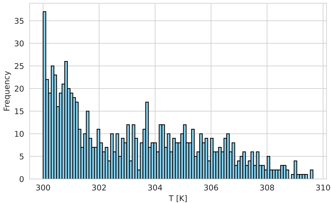
SSP370 Scenario
