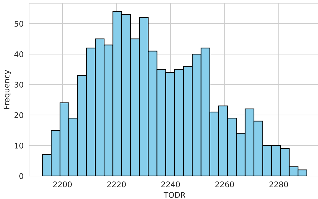
SSP370 Scenario
