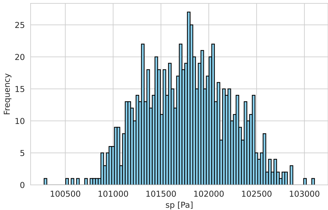
SSP370 Scenario
