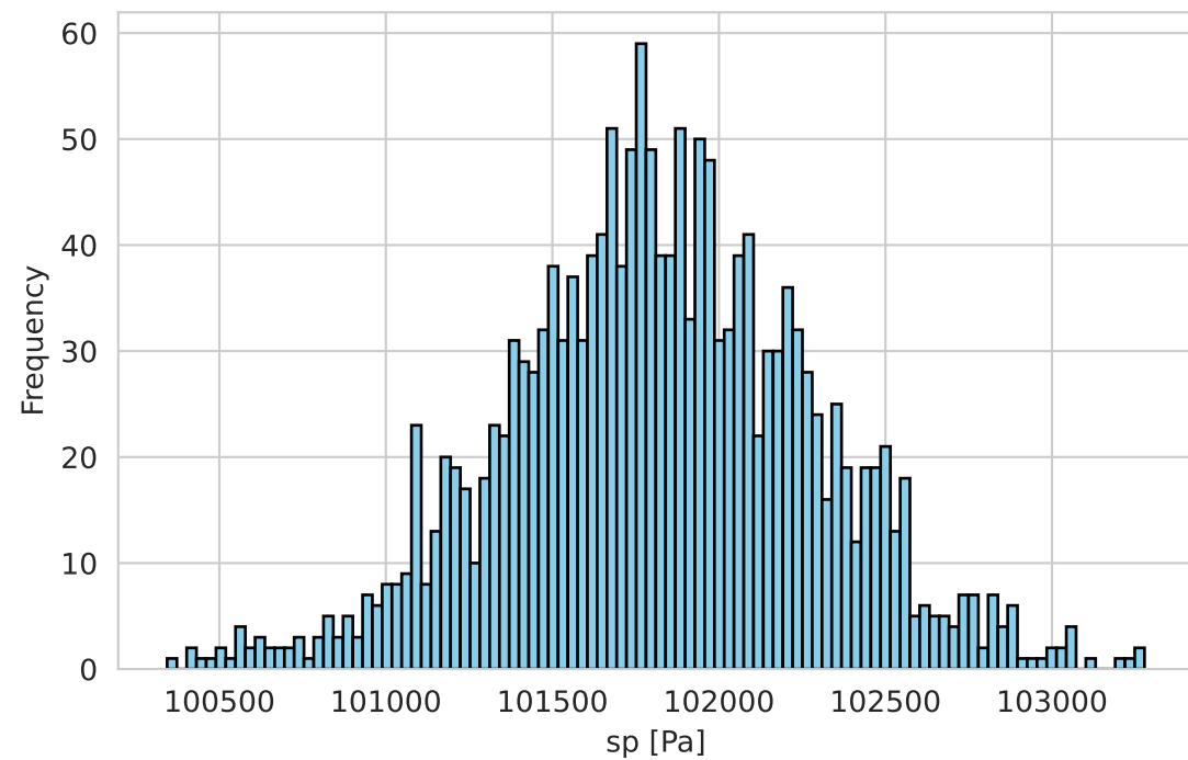
SSP585 Scenario
