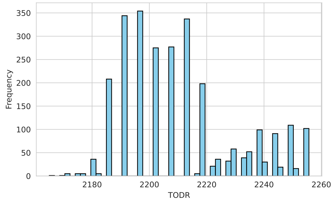
SSP585 Scenario
