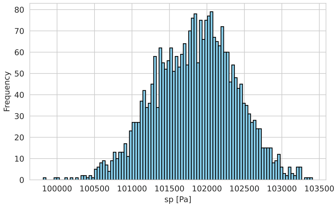
SSP370 Scenario
