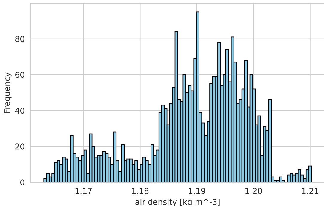
SSP370 Scenario
