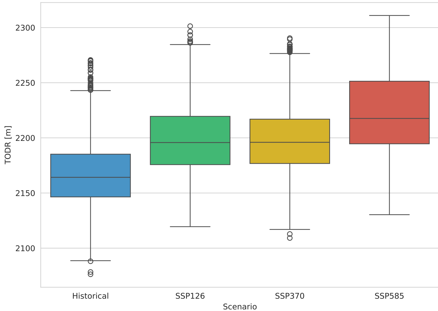
TODR (IIA) A320 - V2500-A1 - EBBR - NOQDM
