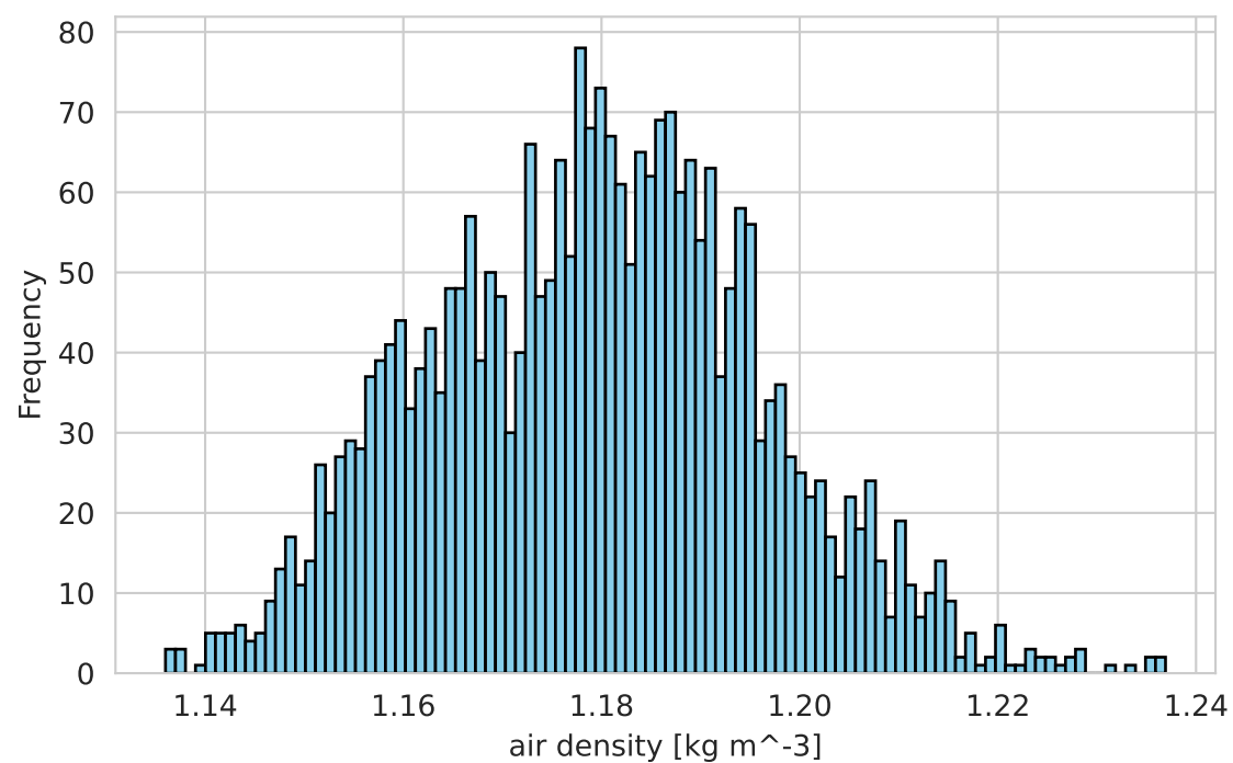
SSP585 Scenario
