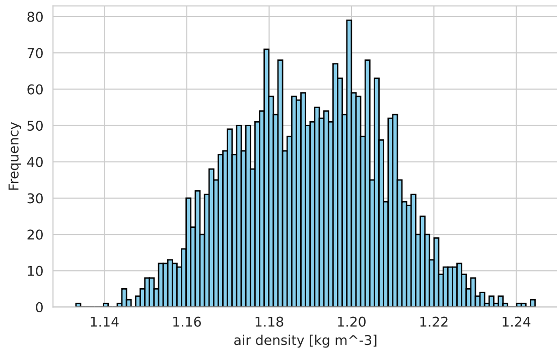
SSP585 Scenario
