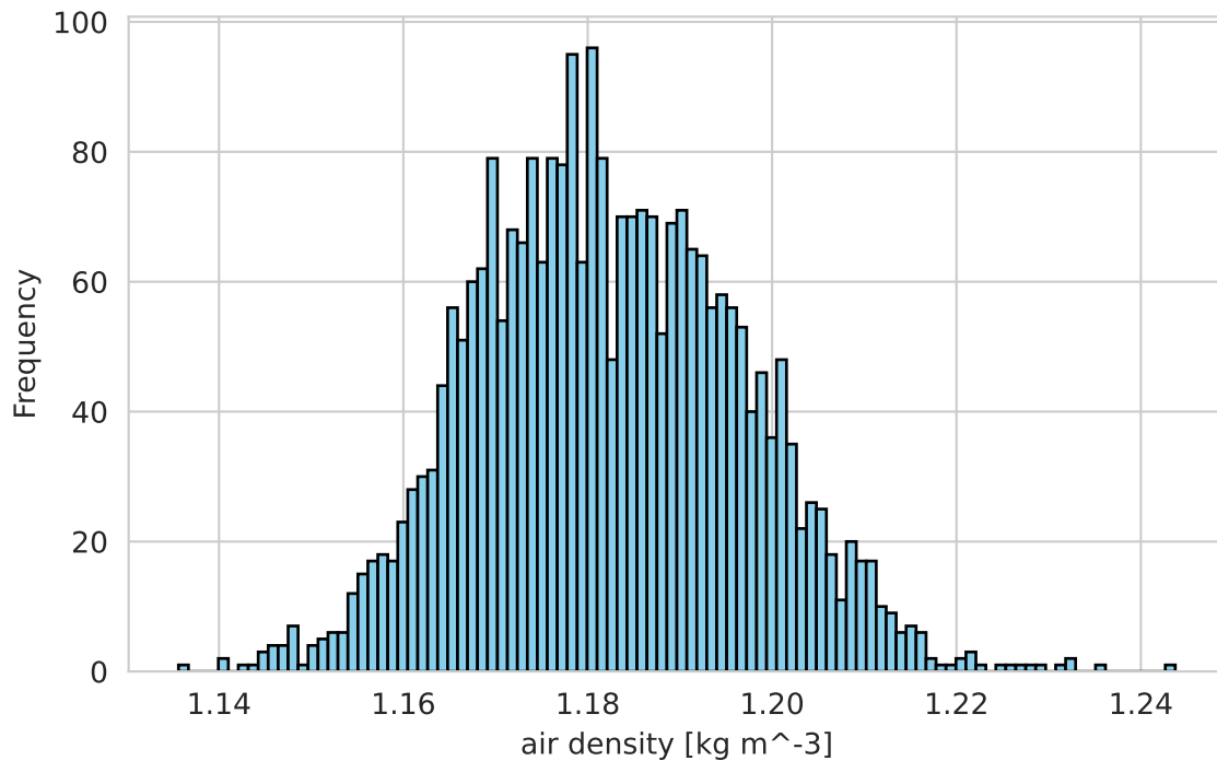
SSP370 Scenario
