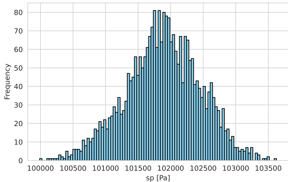
SSP585 Scenario
