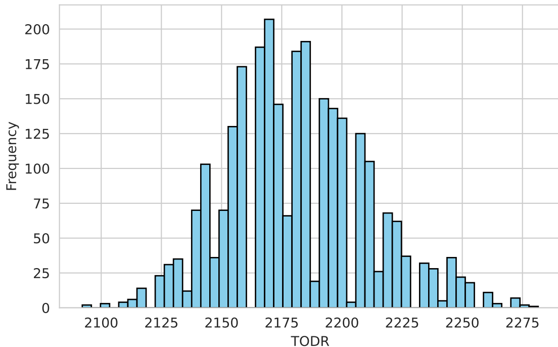
SSP370 Scenario
