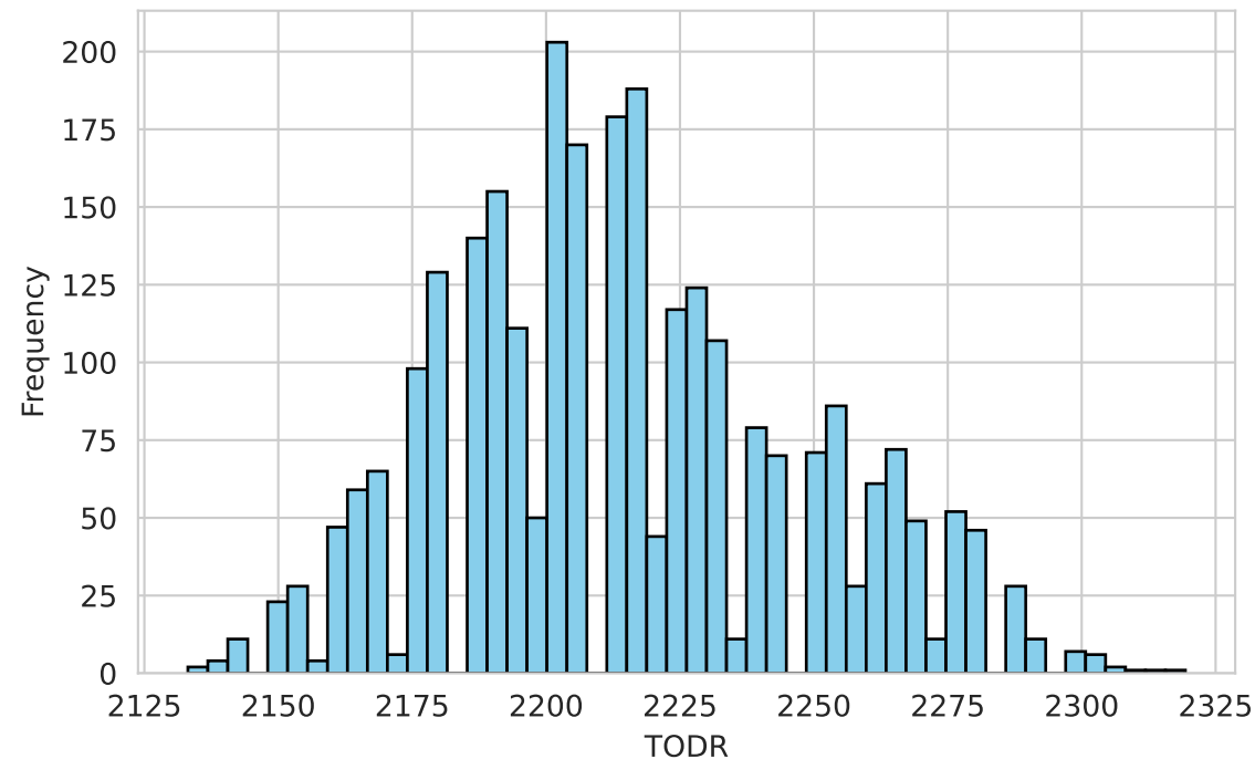
SSP585 Scenario
