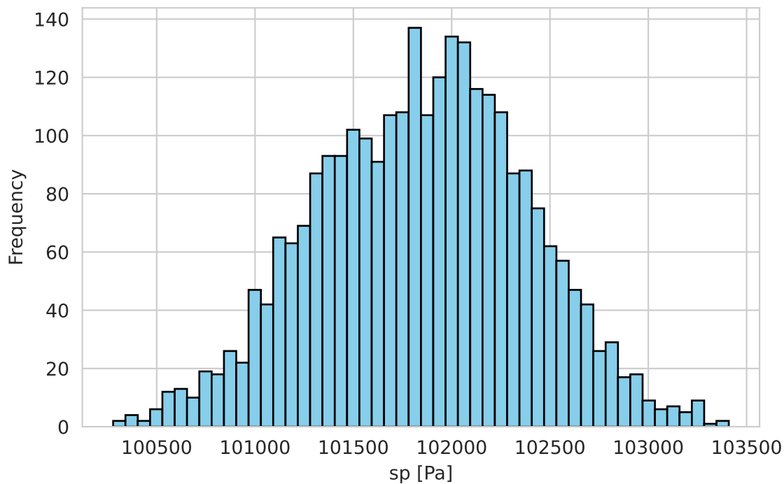
SSP370 Scenario
