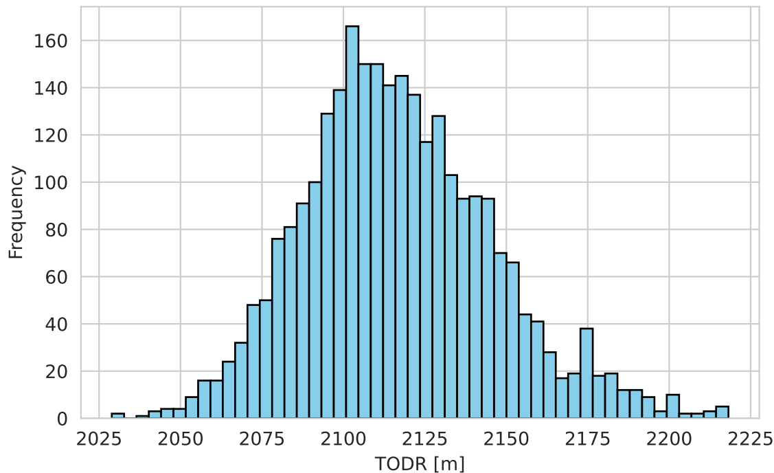
SSP370 Scenario
