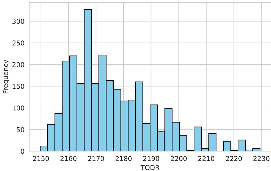
SSP370 Scenario
