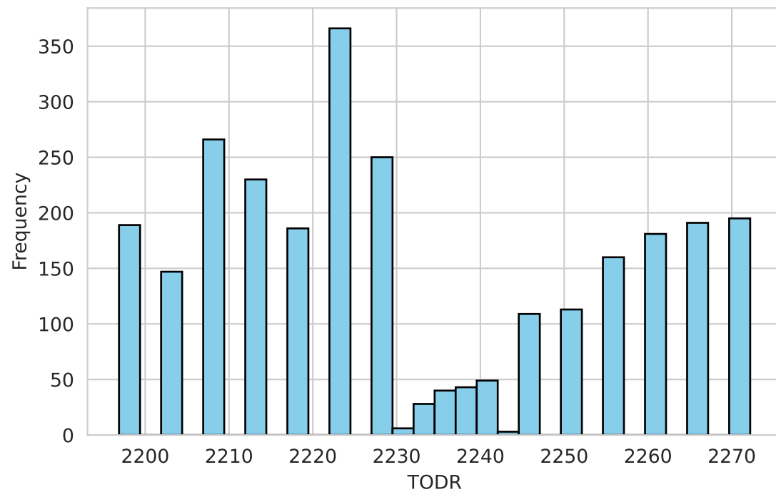
SSP585 Scenario
