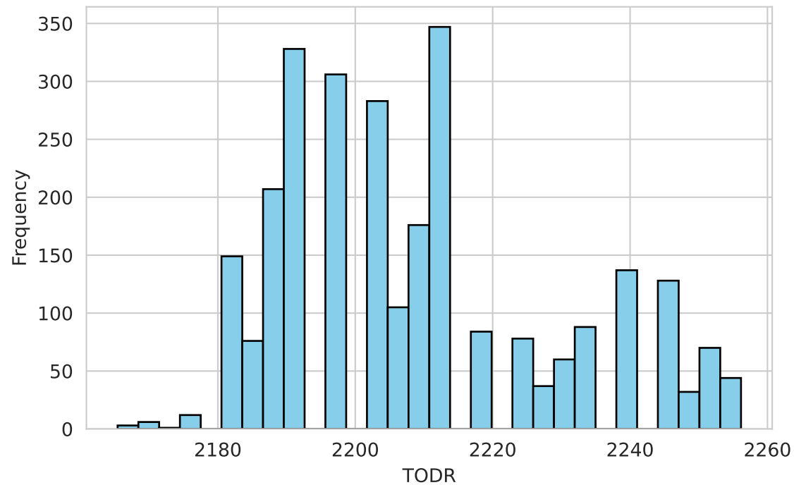
SSP585 Scenario
