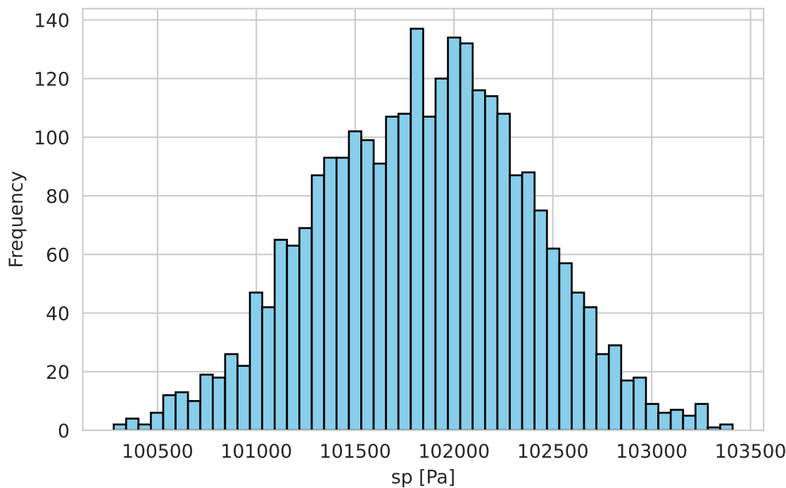
SSP370 Scenario
