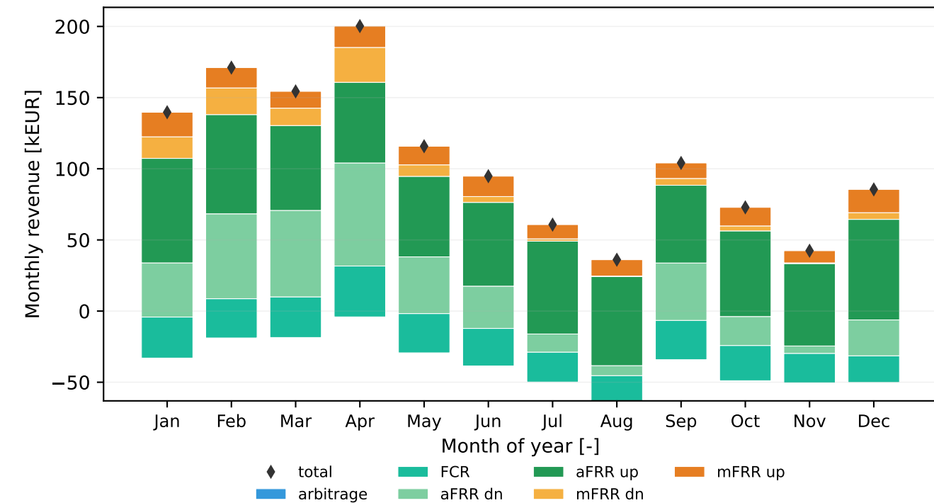
PPO vanilla
