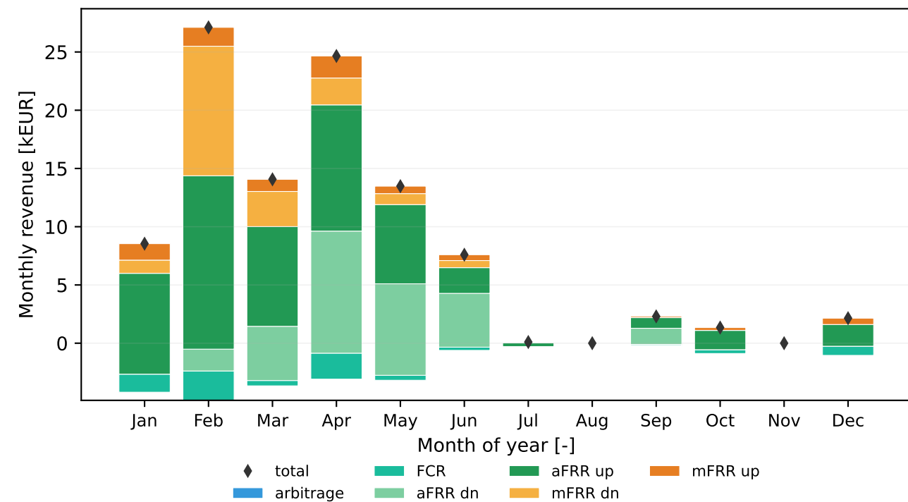
PPO vanilla
