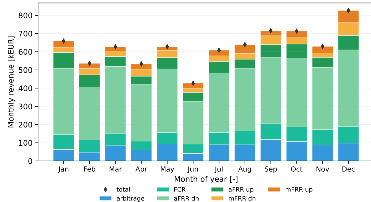
PPO vanilla
