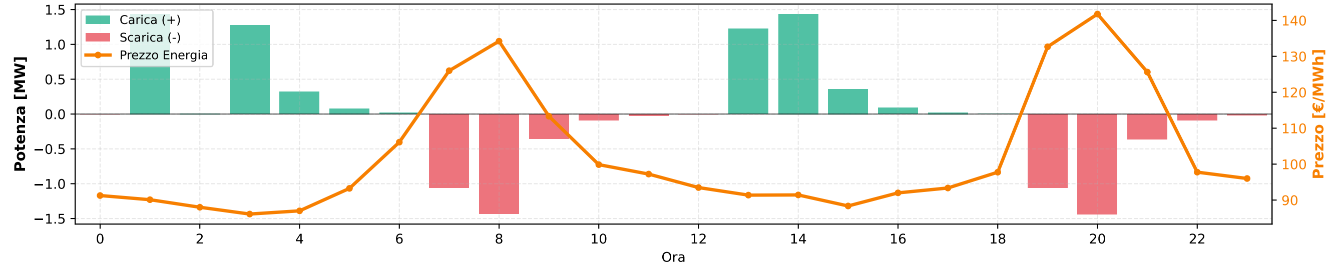
Potenza BESS e Prezzo Energia
