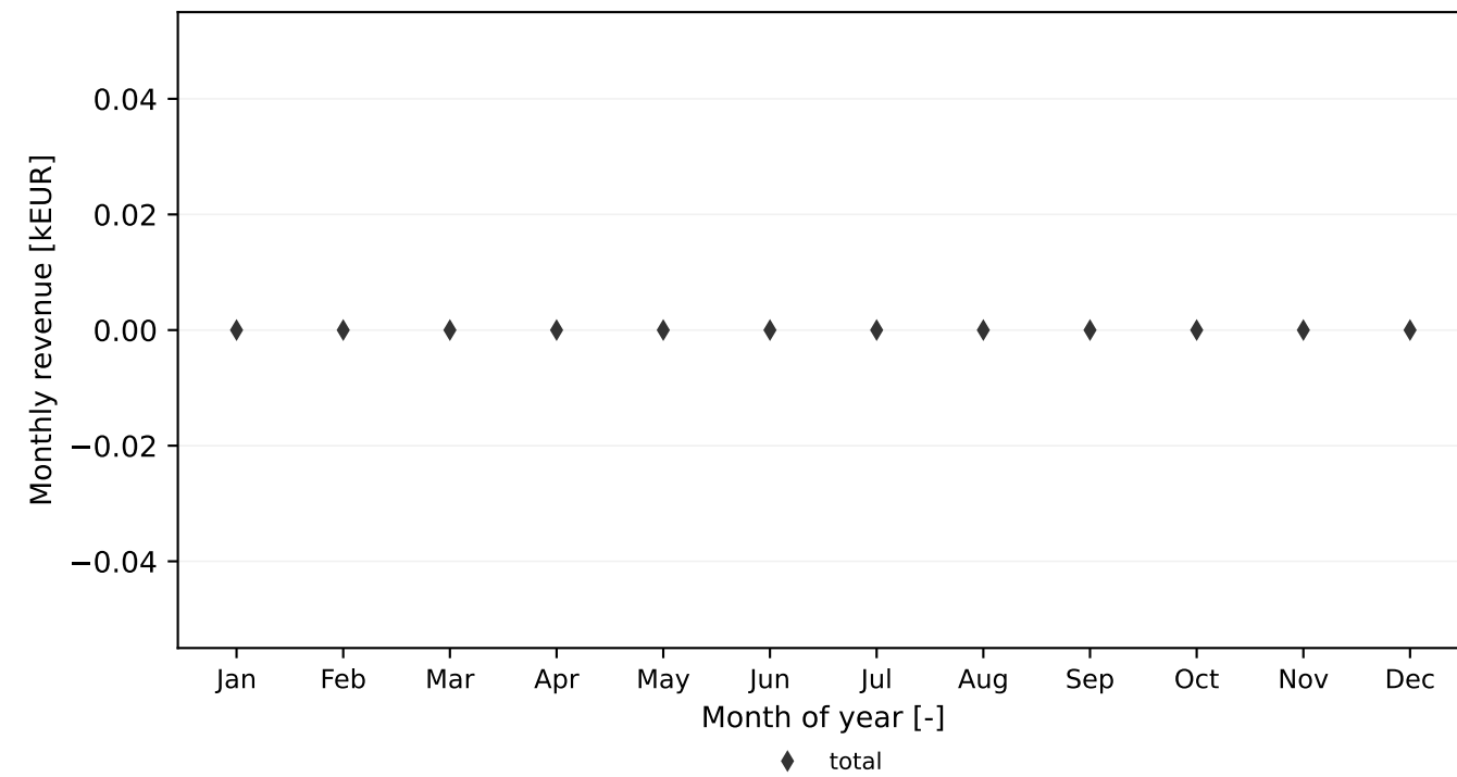
PPO vanilla
