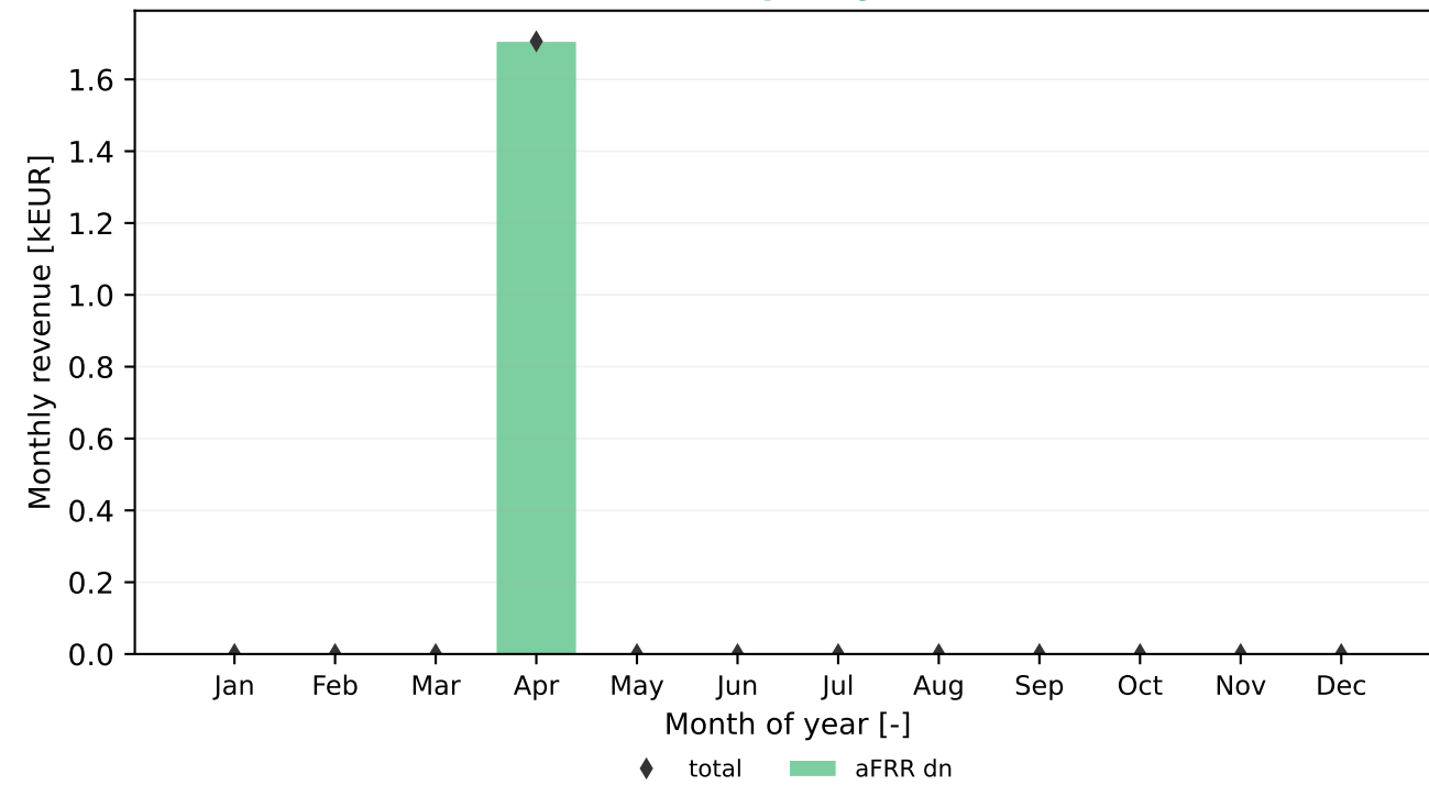
PPO vanilla
