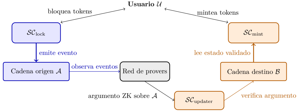
Fig. 2.1: Esquema operativo de un zkBridge entre una cadena origen \mathcal{A} y una cadena destino \mathcal{B} . El usuario bloquea activos en \mathcal{SC}_{\text{lock}} , una red de provers observa el evento y genera un argumento ZK sobre el estado de \mathcal{A} , el contrato \mathcal{SC}_{\text{updater}} verifica ese argumento en \mathcal{B} , y el contrato \mathcal{SC}_{\text{mint}} usa el estado autenticado para emitir los activos envueltos.
