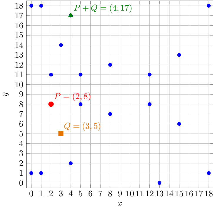
Fig. A.4: Puntos de \mathcal{E}(\mathbb{F}_{19}) para la curva y^2 = x^3 - x + 1 . Los puntos azules son todas las soluciones sobre \mathbb{F}_{19} ; se destacan P = (2, 8) en rojo, Q = (3, 5) en naranja y el resultado de la suma algebraica P + Q = (4, 17) en verde, calculado con las fórmulas de grupo sobre cuerpos finitos.
