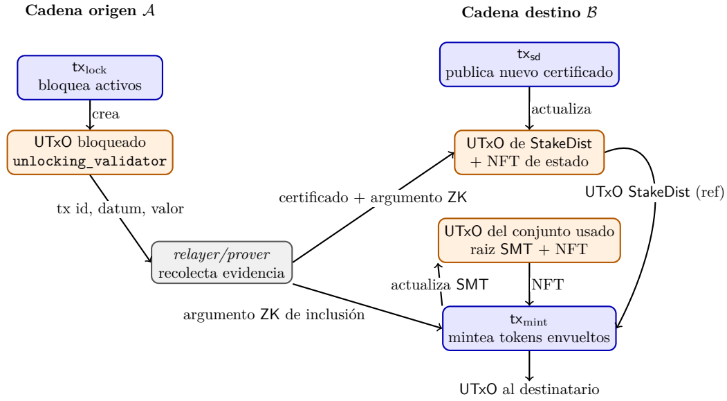
Fig. 5.1: Flujo transaccional de la primera etapa del zkBridge para el camino tx_{lock} \rightarrow tx_{mint} . La tx_{lock} crea un UTxO bloqueado en la cadena origen; el relayer/prover recolecta el identificador, datum, valor y evidencia criptográfica; en la cadena destino, tx_{sd} actualiza el UTxO de StakeDist y tx_{mint} mientea tokens envueltos mientras actualiza el conjunto anti-replay resumido por una raíz SMT.
