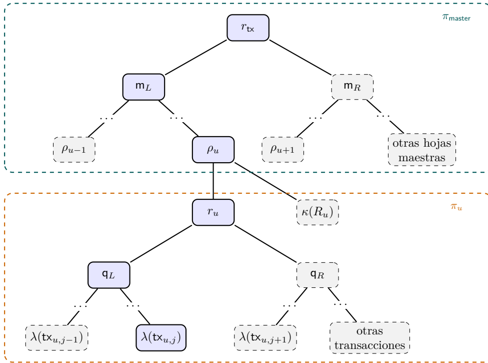
Fig. 6.2: Estructura de una prueba de pertenencia en CardanoTransactions legacy . La \pi_u certifica que una transacción concreta pertenece al Merkle Tree de un rango de bloques R_u ; la \pi_{master} certifica que la hoja maestra \rho_u , formada por \kappa(R_u) y r_u , pertenece al Merkle Tree maestro cuya raíz firmada es r_{tx} .
