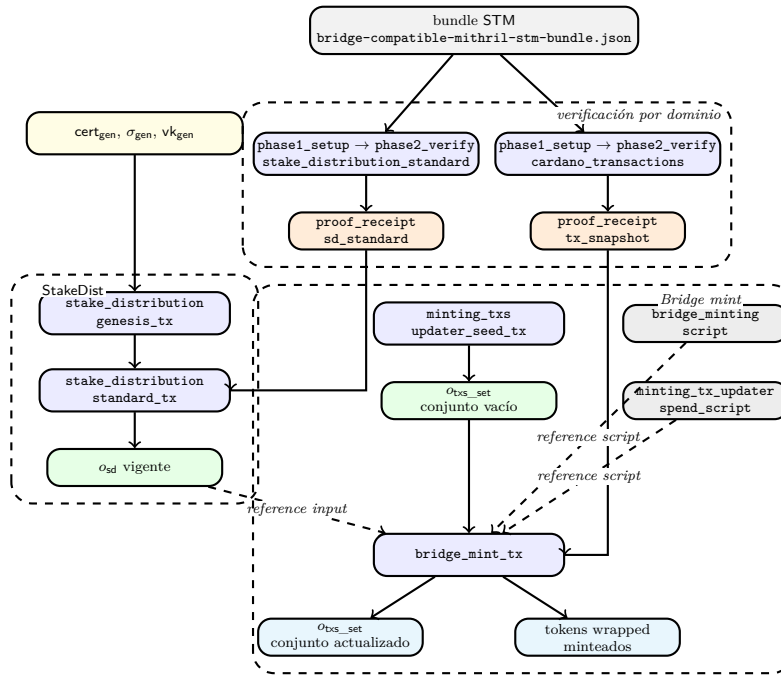
Fig. 7.1: Flujo final implementado del zkBridge. El bundle STM alimenta las dos verificaciones por dominio que producen proof_receipt para stake_distribution_standard y cardano_transactions ; el cert_gen inicializa la cadena de StakeDist sin receipt; la transacción bridge_mint_tx consume el receipt de transacciones y el o_{txs\_set} , usa el o_{sd} como reference input y reutiliza scripts pesados como reference scripts para emitir tokens envueltos y actualizar el conjunto anti-replay.
