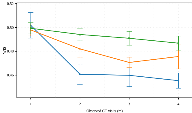
C. Conformal WIS
