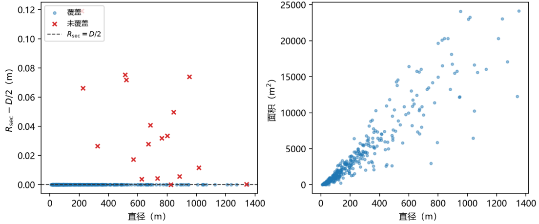
图 7 左：400 个有界样本的残差 R_{\text{sec}} - D/2 ；右：定位多边形面积与直径。
