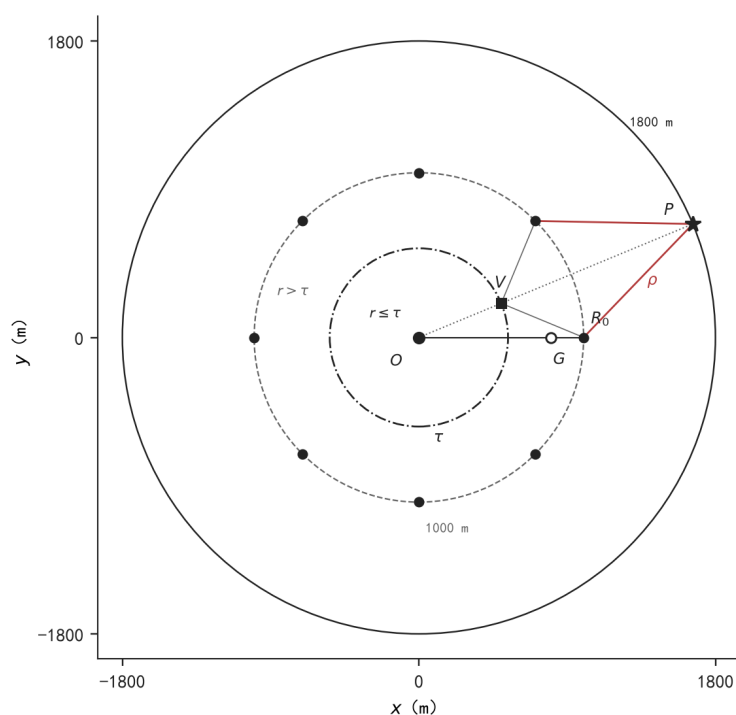
图 13 问题三 9 盘覆盖。实线为场地 1800 m，虚线为环点所在的 1000 m 设计听距圆，点划线为原点-环点等距分界点半径 \tau \approx 541 m。 r \leq \tau 由原点覆盖； r > \tau 由最近环点覆盖，其中 r \in (\tau, 1000] 的最近检测点是环点而不是原点。角平分线上的方点 V 为等距分界点，最远点 P 在场地边界角平分处，红弦为 \rho 。白点 G 落在 (\tau, 1000] 内。线段 OR_0 长 1000 m，故 8 环不能覆盖原点。
