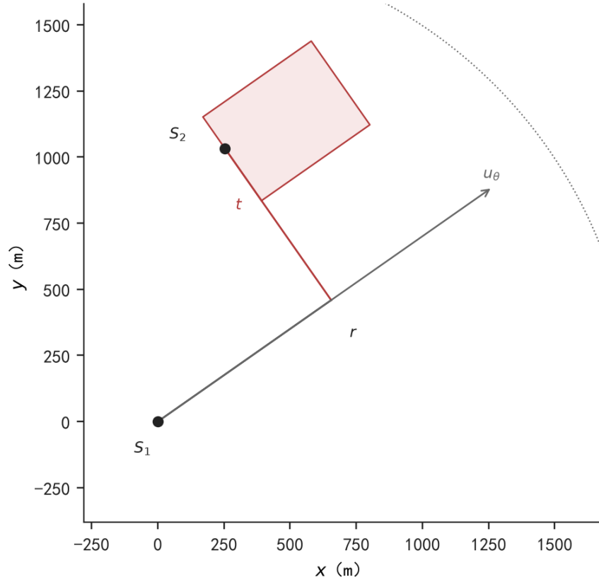
图 8 第二站离开第一示向度轴：轴向距离 r 、横向偏移 t 。第二个检测点在 |t| = 700 m 由轴上 \psi \geq 45^\circ 覆盖给出；比较候选点 |t| = 690.9 m 只作比较。
