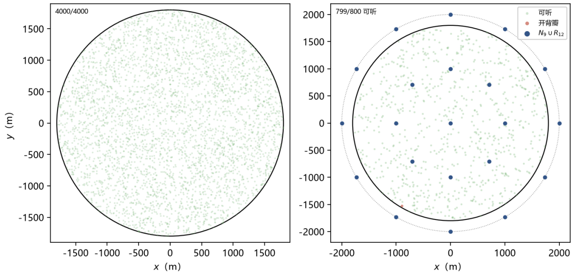
图 18 左：问题三 9 点网的全向覆盖（场地圆盘均匀样本 n = 4000 ，未覆盖点不出现）；右：问题四检测网 N_9 \cup R_{12} 上 800 个位置-朝向样本，绿色为可听、红色为背面听不到的一侧残留。该图是抽样核对，不是 \forall u 覆盖定理。
