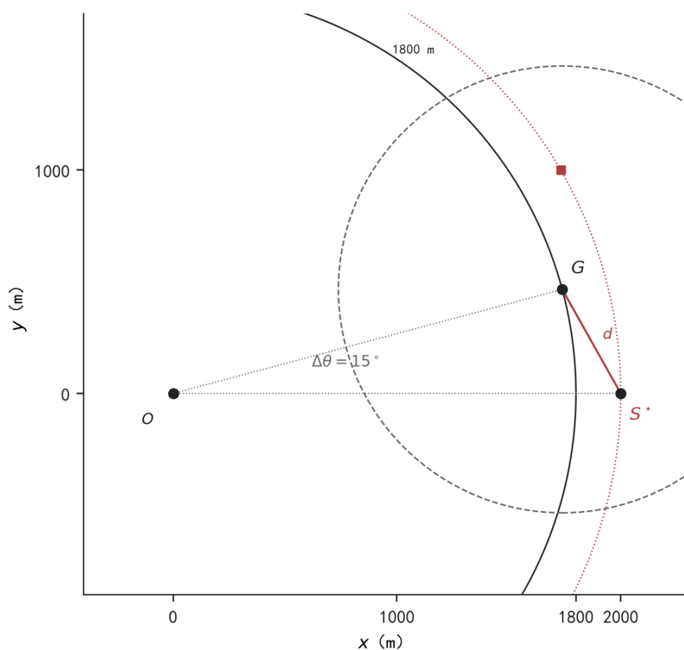
图 22 外环距离引理的中缝剖面： G 在场地边界 1800 \angle 15^\circ ， S^* 在 2000 \angle 0^\circ ，弦长 d \approx 534.17 \text{ m} ，虚线圆是以 G 为心的 1000 m 盘。
