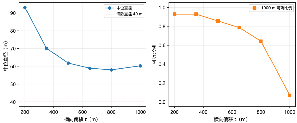
图 11 左：横向偏移对中位直径的影响；右：1000 m 可听比例随横向偏移下降。
