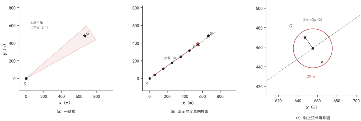
图 17 问题三全向局部化几何。左幅扇形半角为示意放大，正文取 1^\circ ；中幅为覆盖结束后沿测得示向度的单向扩展搜索；右幅轴上 P 满足 \|SP\| = \|SG\| = r ，弦长 2r \sin(|\alpha|/2) ，清除圆半径 20 m。 r \tan 1^\circ 是垂直截面半宽，不是该充要。该图不是发现层的检测点巡查路线，也不表示首次听到的站。
