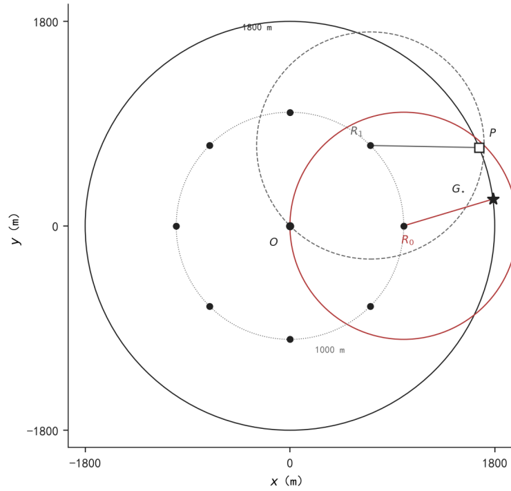
图 14 连续残留与有限样本的差别。红实线圆为 R_0 的 1000 m 盘，红弦连到只被 R_0 听到的 G_* = 1800\angle 7.5^\circ ；灰虚线圆为 R_1 的 1000 m 盘，灰弦连到角平分点 P = 1800\angle 22.5^\circ 。P 可被 R_1 盖住，而 G_* 落在该虚线盘外，仍属 R_0 的独有两圆公共部分。有限角平分点已空不能代替 \text{Res}_{\text{cont}} ，否则会错误跳过 R_0 。
