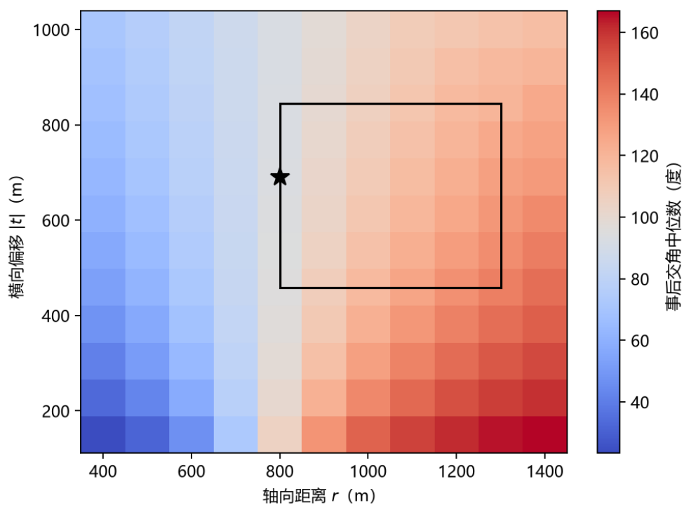
图 10 事后交角中位数随 (r, |t|) 的变化。
