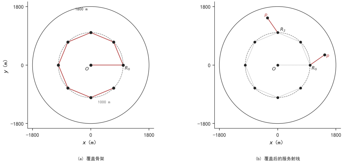
图 16 问题三时间层。左幅检测点巡查路线是原点加 8 环的较短巡查顺序；为缩短时间的走法失败时覆盖义务仍走这 9 网点，不把检测点巡查路线改写成命中即射线的星形。共享 D-最优站可按相对当前路线第一站的路程差抢先作为下一站。右幅一站示向度多数延后到覆盖结束后，接合点取沿测得示向度 550 m 处。两站服务点在覆盖未完时也可进入同一较短巡查顺序，选中后走圆心再测与射线归航。
