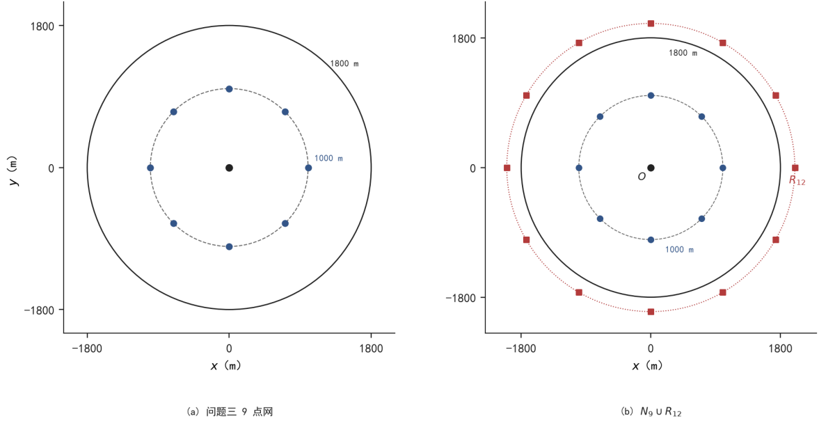
图 15 左：问题三的 9 点检测点组（点在 1000 m 圆上）；右：问题四检测网 N_9 \cup R_{12} ，外环 12 个方点在半径 2000 m 的圆上。
