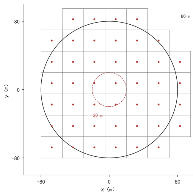
图 24 光学方格可以保证清除的条件：边长 25 m 的闭正方形外接半径约 17.68 m，小于清除半径 20 m；实线盘半径 80 m 是启用该充分条件的限度。
