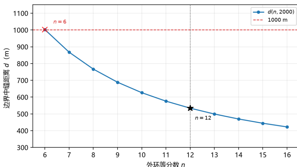
图 26 外环边界中缝距离随等分数的变化。水平虚线为 1000 m；星号为交付 n = 12 ，叉号为不合格 n = 6 。
