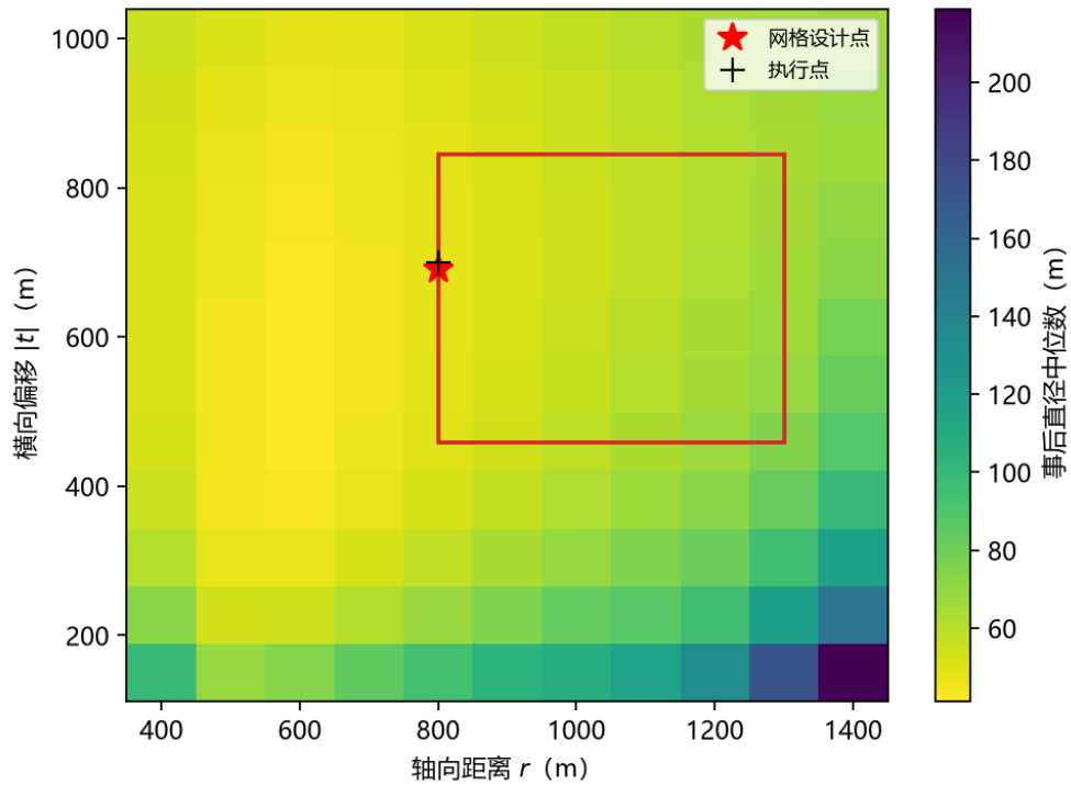
图 13 事后直径中位数随 (r, |t|) 的变化。红框为比较带，星号为网格分位点；交付点在 |t| = 700 m。
