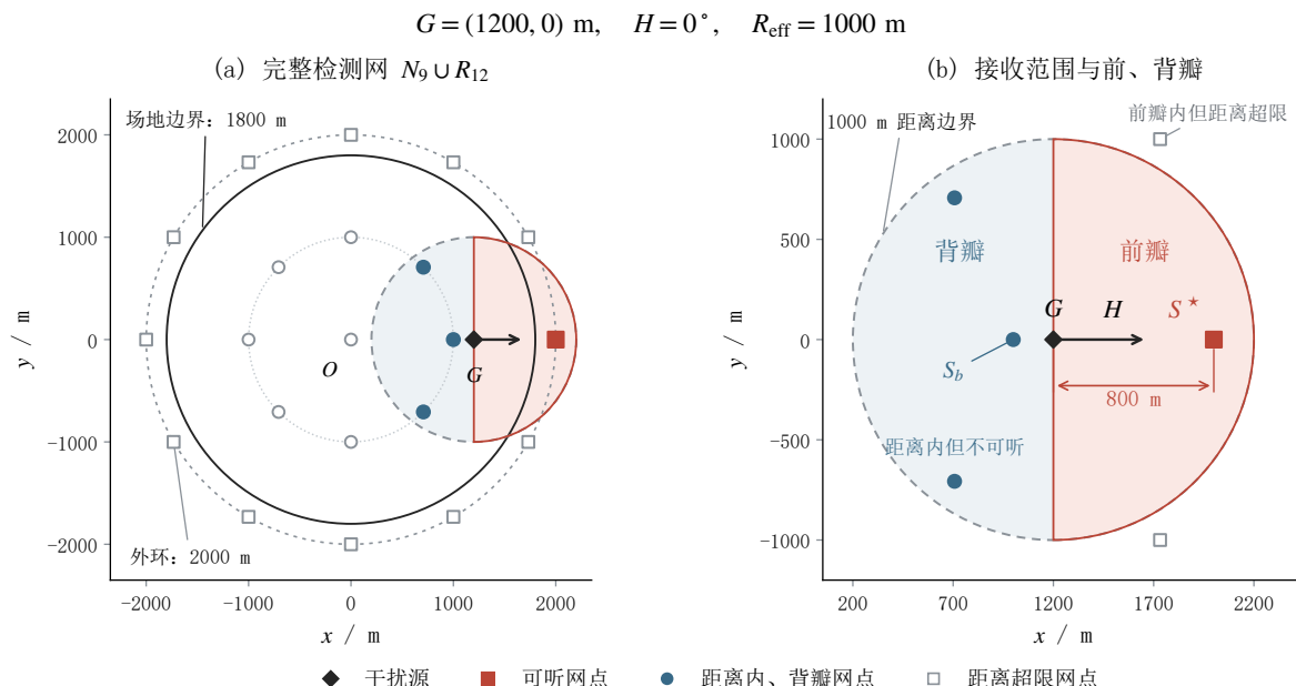
图 24 定向源的距离与朝向联合判定 ( R_{\text{eff}} = 1000\text{ m} )。左：完整检测网，圆点、方点分别为 N_9 、 R_{12} ，黑实线为场地边界。右： G = (1200, 0)\text{ m} ，朝向正东；红点 S^* = (2000, 0)\text{ m} 距源 800\text{ m} 且在前瓣内，可听。蓝点处于距离盘内的背瓣，其中 S_b 距源仅 200\text{ m} ，仍不可听；灰色空心点距离超限。
