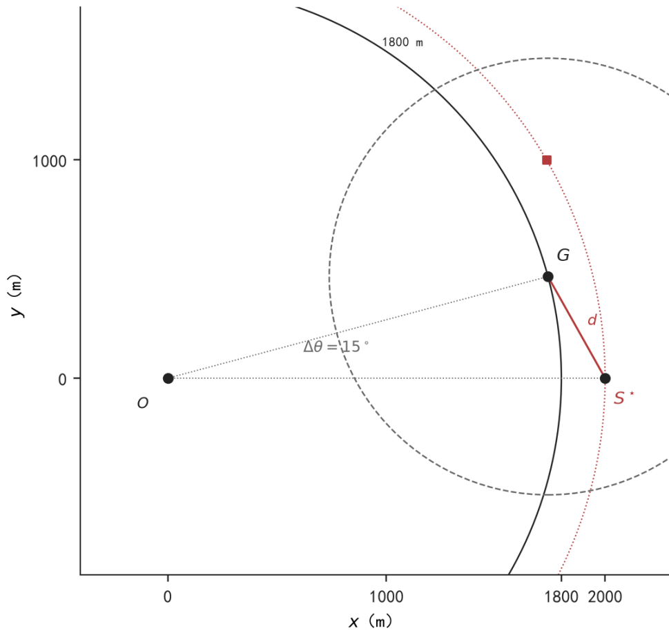
图 26 外环距离引理的中缝剖面：$G$ 在场地边界 $1800\angle 15^\circ$，$S^*$ 在 $2000\angle 0^\circ$，弦长 $d \approx 534.17$ m，虚线圆是以 $G$ 为心的 $1000$ m 盘。
