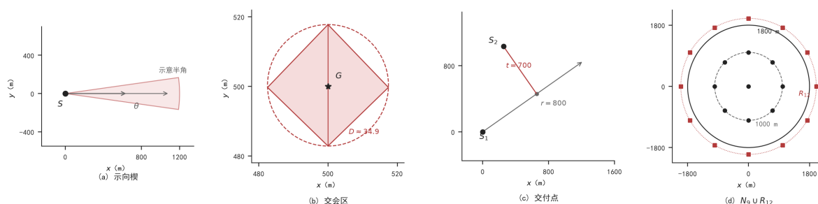
图 1 四问几何衔接。(a) 示向楔（半角为示意放大，正文取 1^\circ ）；(b) 交会区与对径圆；(c) 交付点 (r, t) = (800, 700) \text{ m} ，不是网格分位点 |t| = 690.9 \text{ m} ；(d) 问题四检测网 N_9 \cup R_{12} ，虚线为 1000 m，实线为 1800 m，外环在 2000 m。
