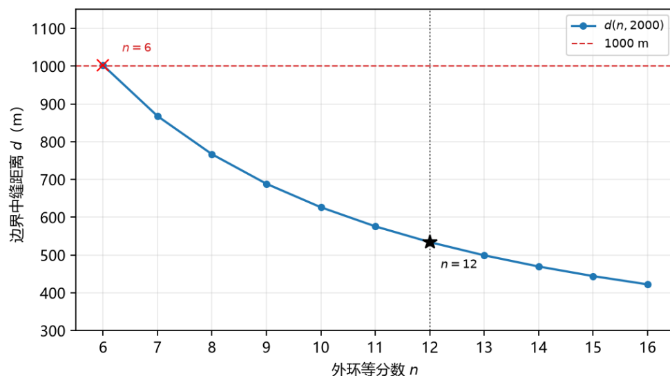
图 30 外环边界中缝距离随等分数的变化。水平虚线为 1000 m; 星号为交付 n = 12 , 叉号为不合格 n = 6 。
