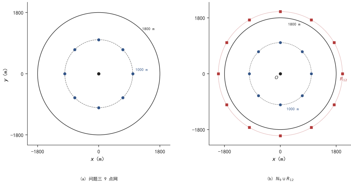
图 19 左：问题三的 9 点检测点组（点在 1000 m 圆上）；右：问题四检测网 N_9 \cup R_{12} ，外环 12 个方点在半径 2000 m 的圆上。
