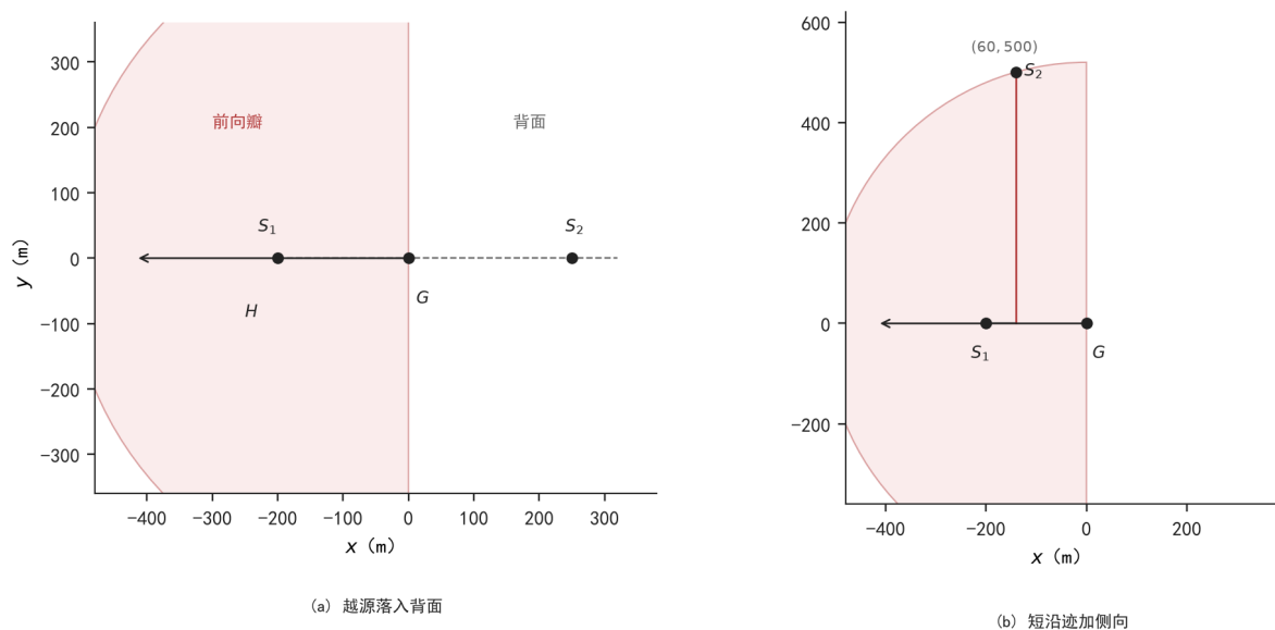
图 27 沿示向度再偏开一点第二站。朝向 H 指向 S_1 所在半平面。左：沿示向度越过源，落入背面；右： (r, t) = (60, 500) m 留在同一闭扇形内。
