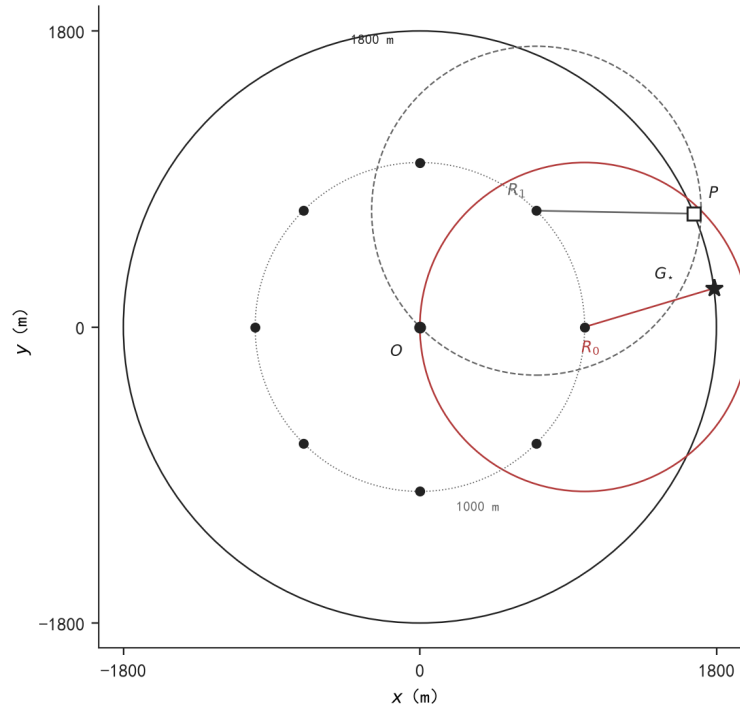
图 18 连续残留与有限样本的差别。红实线圆为 R_0 的 1000 m 盘，红弦连到只被 R_0 听到的 G_* = 1800\angle 7.5^\circ ；灰虚线圆为 R_1 的 1000 m 盘，灰弦连到角平分点 P = 1800\angle 22.5^\circ 。P 可被 R_1 盖住，而 G_* 落在该虚线盘外，仍属 R_0 的独有两圆公共部分。有限角平分点已空不能代替 \text{Res}_{\text{cont}} ，否则会错误跳过 R_0 。
