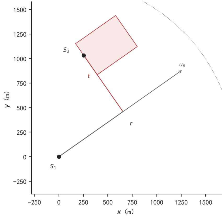
图 12 第二站离开第一示向度轴：轴向距离 r 、横向偏移 t 。第二个检测点在 |t| = 700 m 由轴上 \psi \geq 45^\circ 覆盖给出；比较候选点 |t| = 690.9 m 只作比较。
