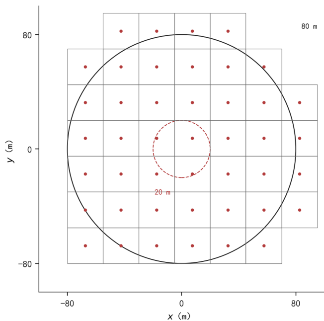
图 28 光学方格可以保证清除的条件：边长 25 m 的闭正方形外接半径约 17.68 m，小于清除半径 20 m；实线盘半径 80 m 是启用该充分条件的限度。
