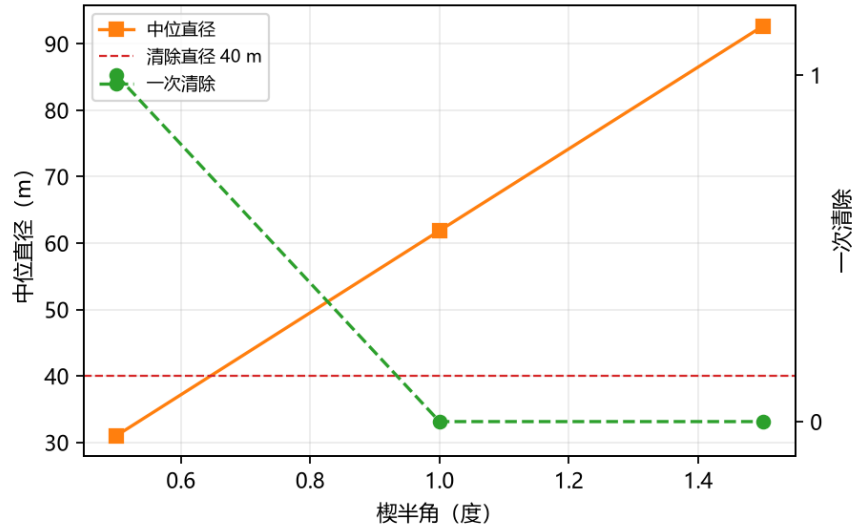
图 16 扇形半角对中位直径与一次清除的影响，剖面 (r, t) = (1100, 500) m。橙实线为中位直径，绿虚线为一次清除，红虚线为清除直径 40 m。
