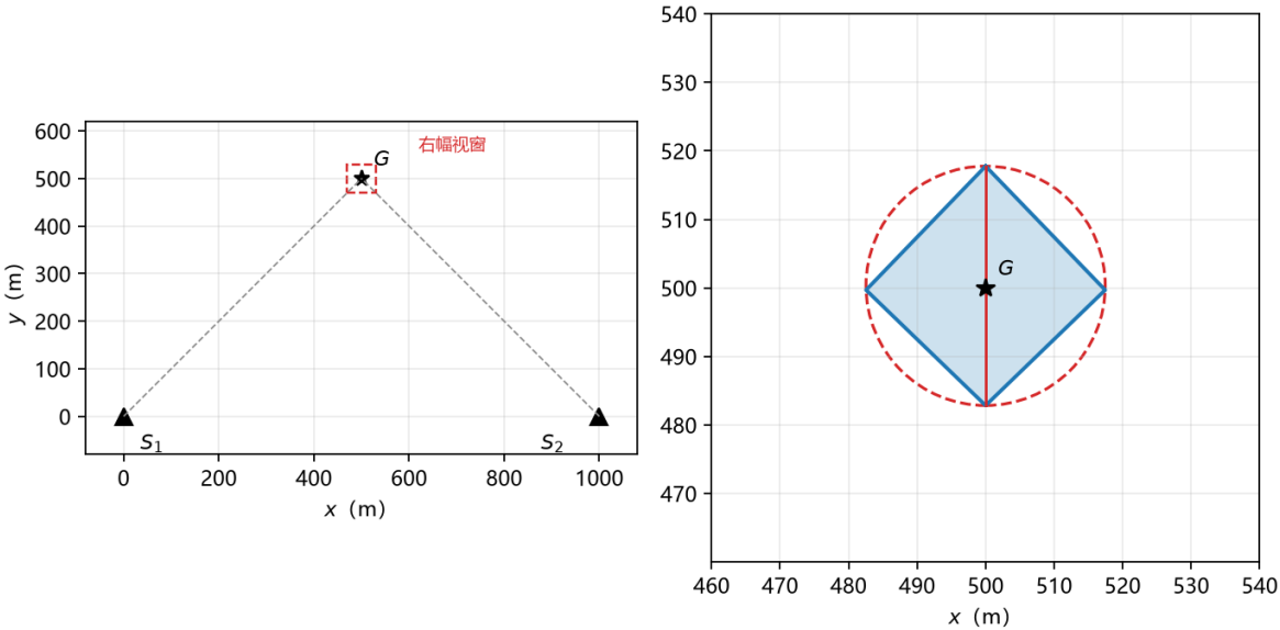
图 9 正交交会合成例。左：两站与真源；右：定位四边形及其以直径为直径的圆。
