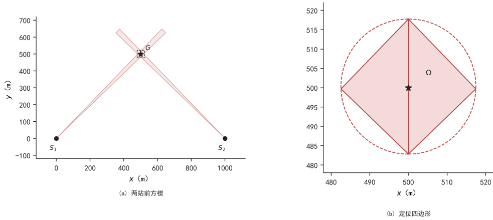
图 7 两站前方扇形之交构成定位区域 \Omega 。左：真半角 1^\circ ；右：交会区放大。
