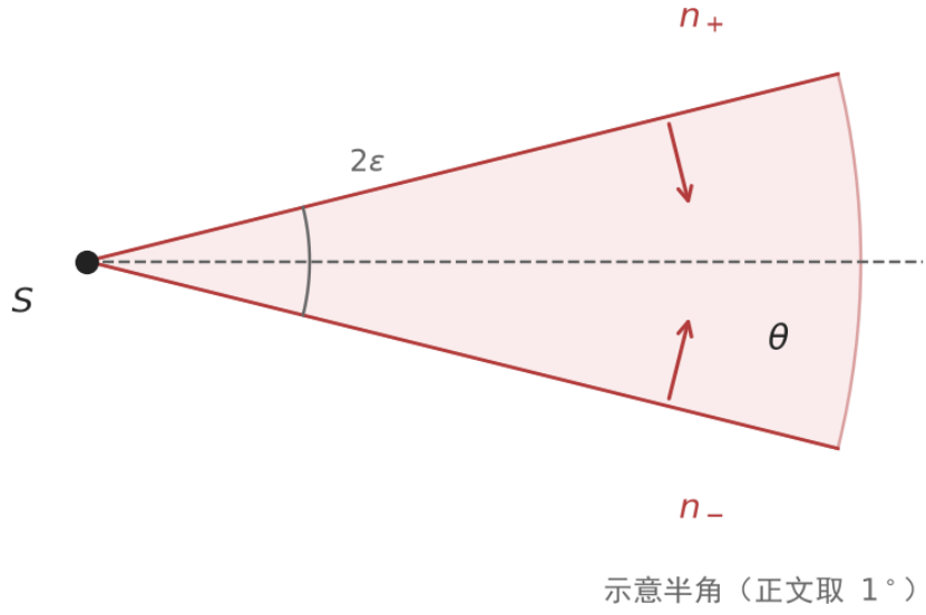
图 6 单站示向度扇形：轴为 \theta ，左右边界的内法向为 n_+ 与 n_- 。
