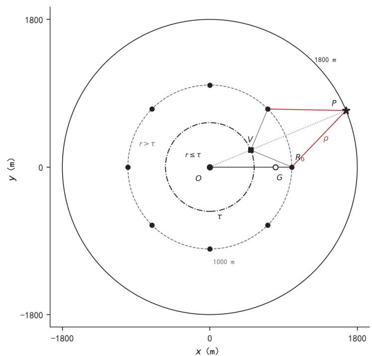
图 17 问题三 9 盘覆盖。实线为场地 1800 m，虚线为环点所在的 1000 m 设计听距圆，点划线为原点-环点等距分界点半径 \tau \approx 541 m。 r \leq \tau 由原点覆盖； r > \tau 由最近环点覆盖，其中 r \in (\tau, 1000] 的最近检测点是环点而不是原点。角平分线上的方点 V 为等距分界点，最远点 P 在场地边界角平分处，红弦为 \rho 。白点 G 落在 (\tau, 1000] 内。线段 OR_0 长 1000 m，故 8 环不能覆盖原点。
