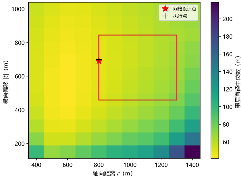
图 13 事后直径中位数随 (r, |t|) 的变化。红框为比较带，星号为比较候选点；第二个检测点 (800, 700) m 在 |t| = 700 m。
