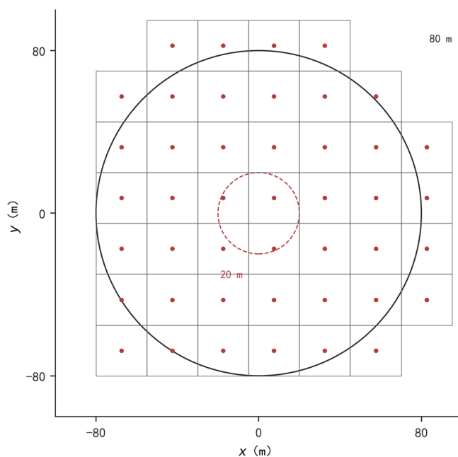
图 24 光学方格可以保证清除的条件：边长 25 \text{ m} 的闭正方形外接半径约 17.68 \text{ m} ，小于清除半径 20 \text{ m} ；实线盘半径 80 \text{ m} 是启用该充分条件的限度。
