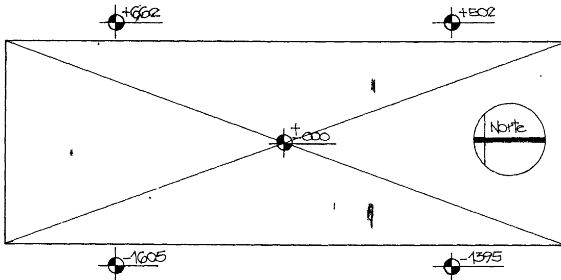
PLANTA NIVELACION
