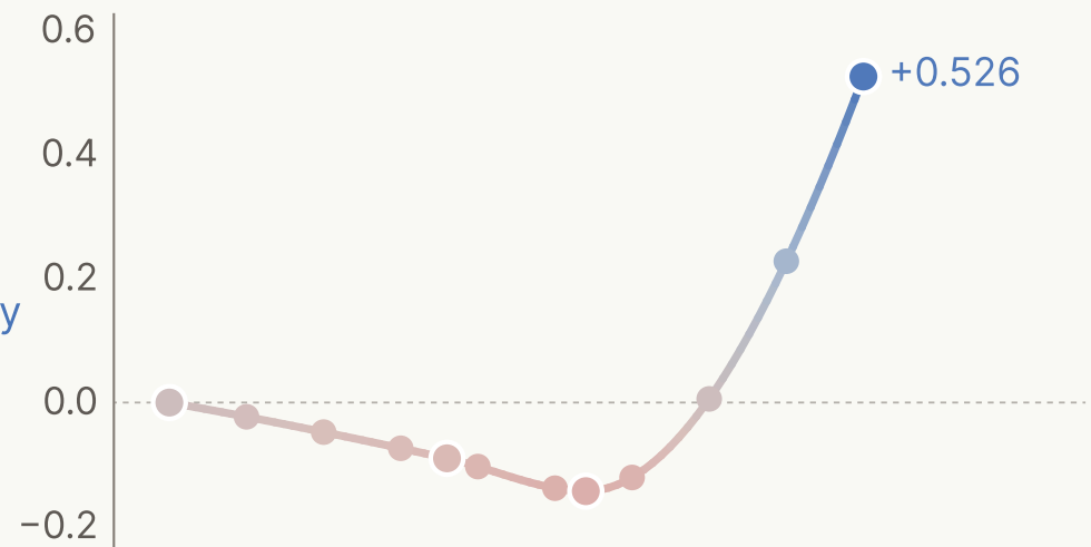
GPT-OSS
