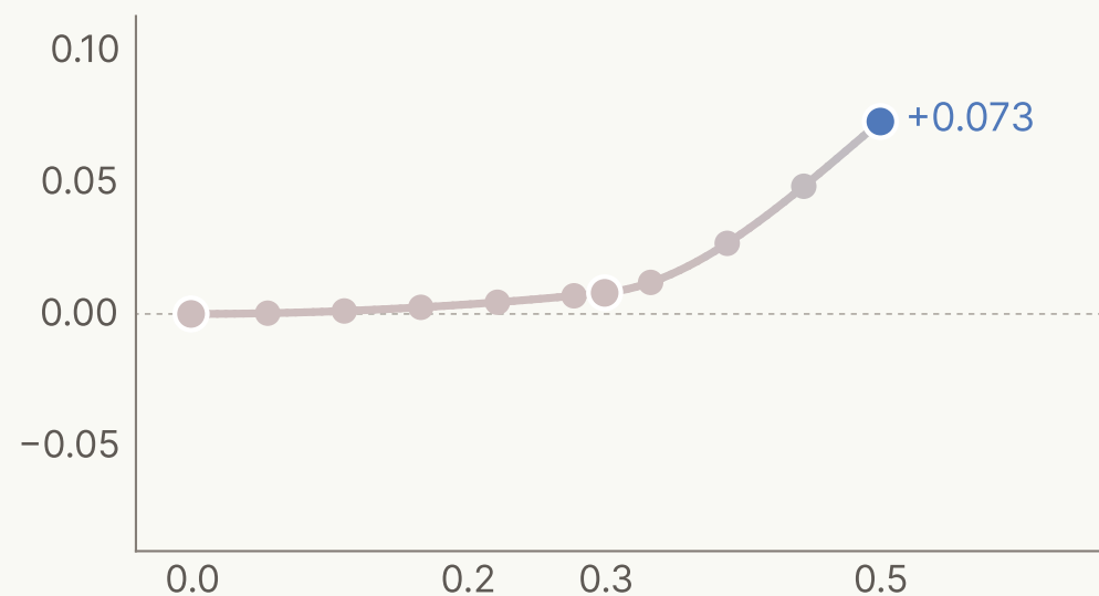
OLMo-2
