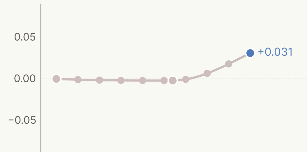
Gemma-4
