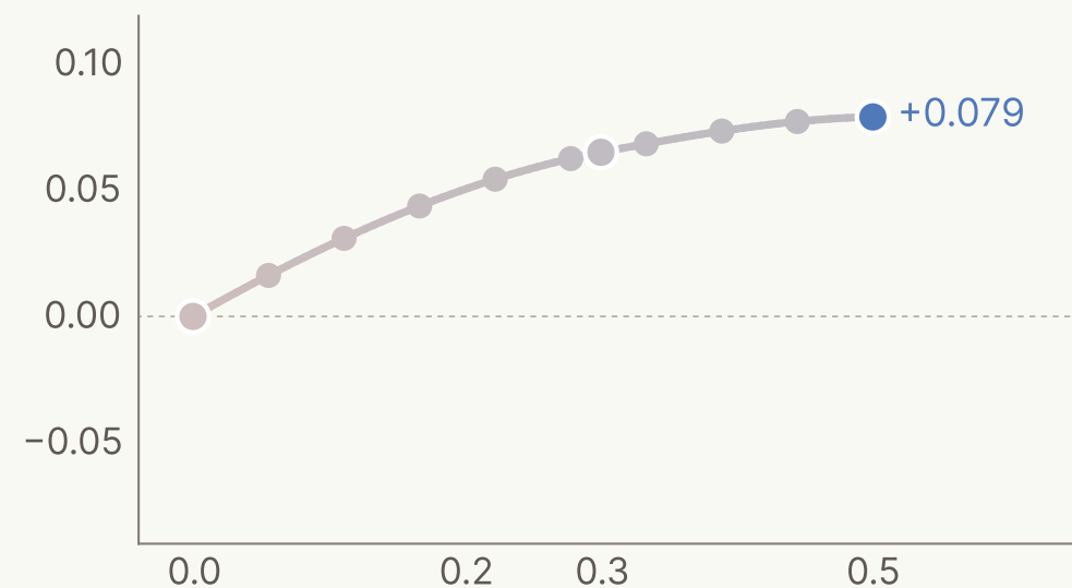
OLMo-3.1
