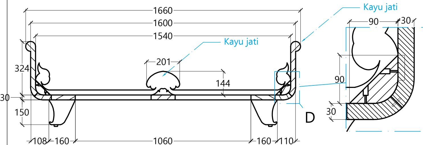
section A'
