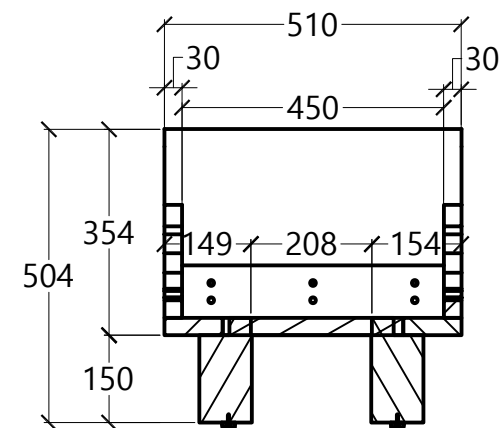
section B'
