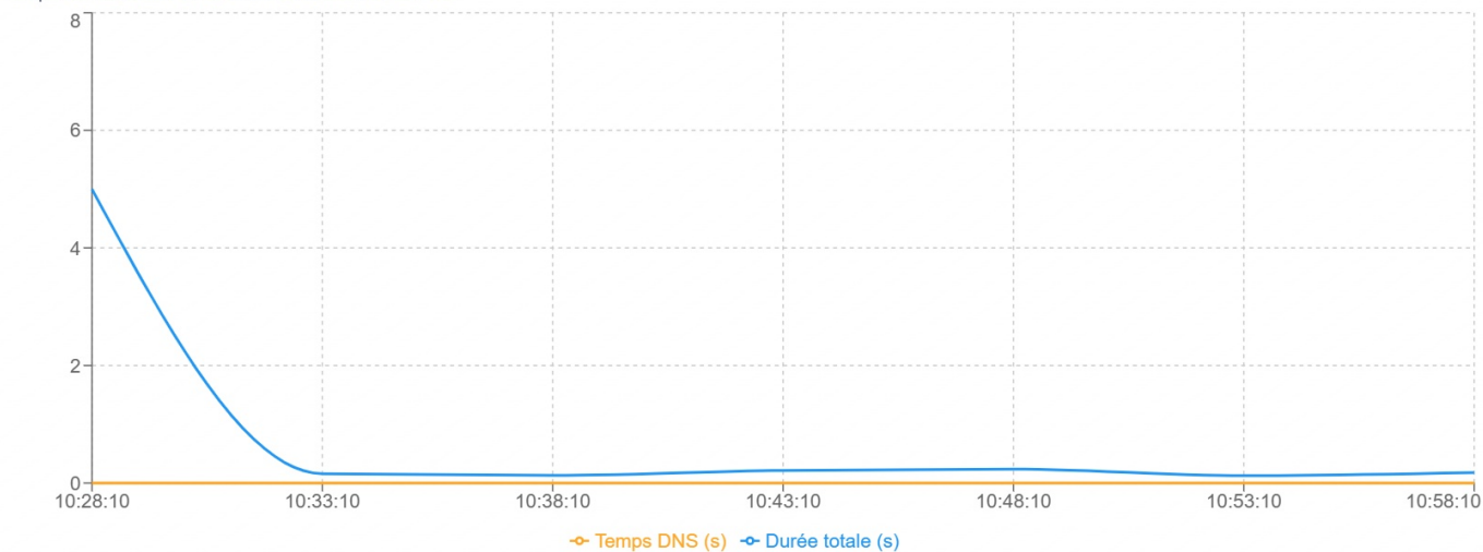
Temps de résolution DNS et durée totale des sondes
