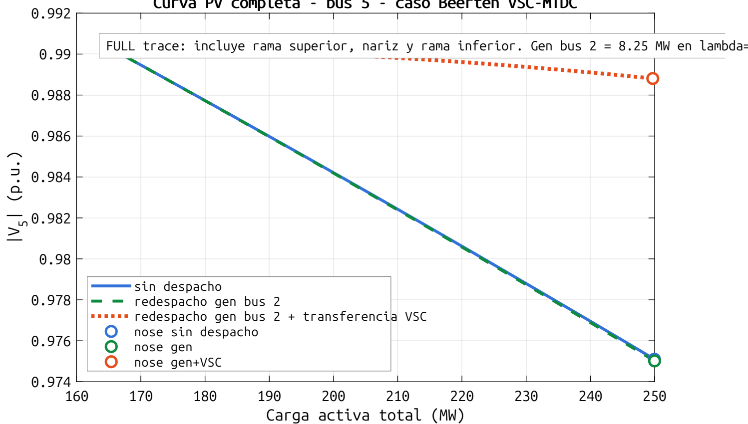
Curva PV completa - bus 5 - caso Beerten VSC-MTDC
