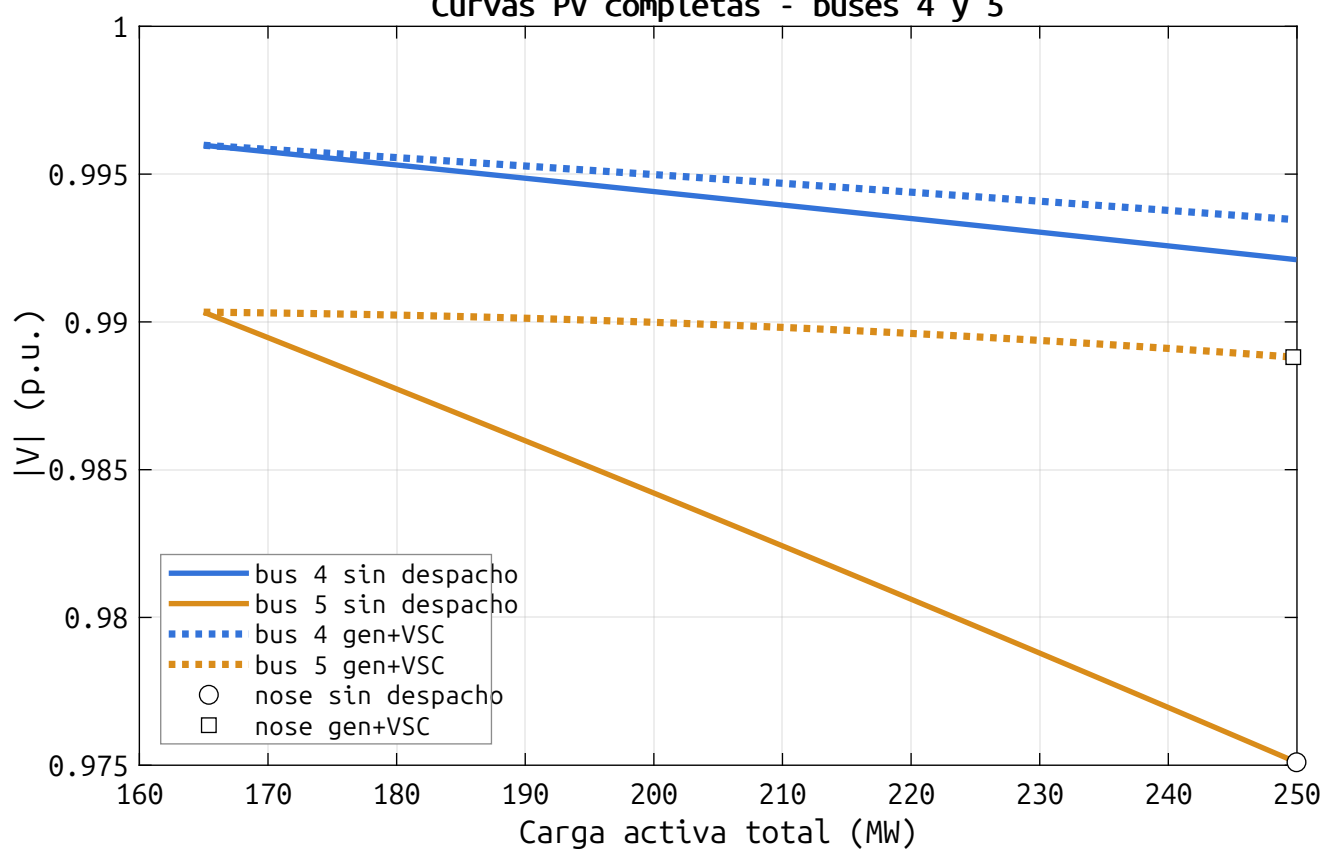
Curvas PV completas - buses 4 y 5
